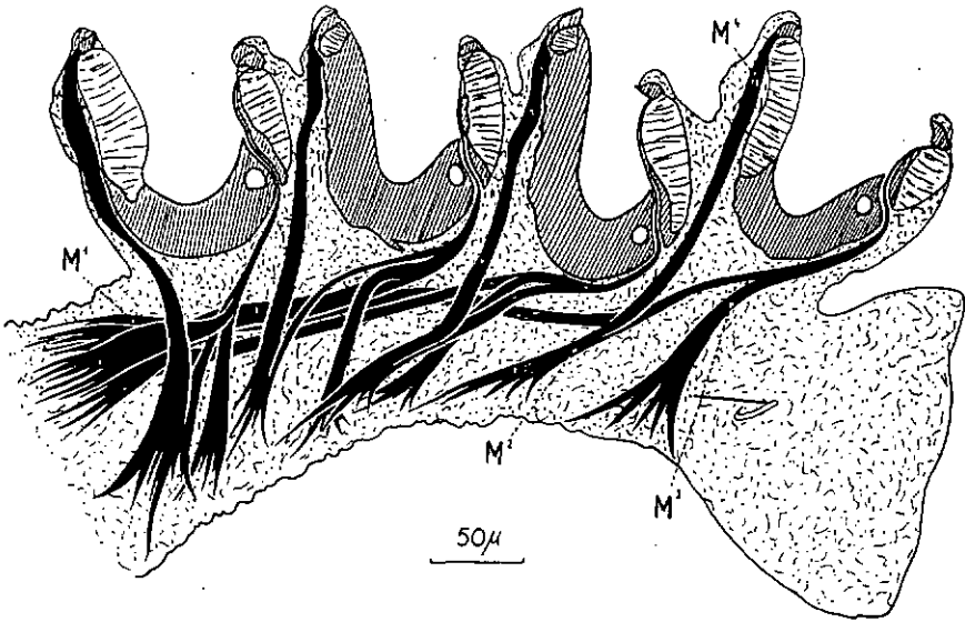
Fig. 5. Semi-schématiquement : détail de la musculature médiane d'une rangée de pincés obtenu par reconstitution à partir de coupes sèriées sagittales du haptcur. (Rangée droite d'un Ver adulte de Vengeron : vue latèrale de l'extèrieur vers l'intèrieur du Ver.) M 1 , M 2 , M 3 et M 4 : branches musculaires médianes de la 1 re pince. Au niveau des pincés ne figurent que les coupes montrant le cheminement du tendon.
