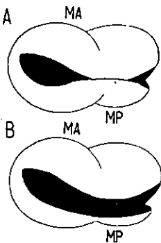
Fig. 6. A : pince fermée montrant latéralement les deux orifices maintenus ouverts par la sclérite C (voir le texte) ; B : pince ouverte ; MA : mâchoire antérieure ; MP : mâchoire postérieure.
