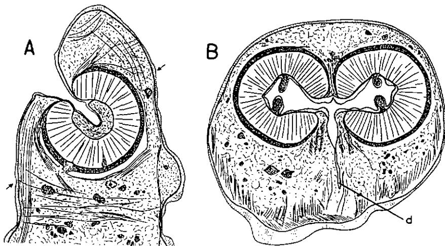
Fig. 14. A : coupe sagittale au niveau d'un organe buccal, passant par l'épaissement en fer à cheval. Au-dessous, légèrement à gauche, une connexion nerveuse se rendant au tissu prismatique. Les flèches indiquent le plan de coupe, en B. B : coupe oblique antéro-postérieure de la région céphalique au niveau des organes buccaux. On distingue ventralement le passage du vestibule péripharyngien à la cavité buccale. — d : extrémité supérieure du canal bucco-intestinal.
