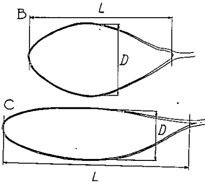
Fig. 39. Méthode de mesure des œufs. B : œuf de la forme inféodée au Vengeron ; C : œuf de la forme inféodée à la Brême ; L : longueur ; D : diamètre. (Les lettres B et C correspondent à celles de la fig. 41. Voir le texte.)
