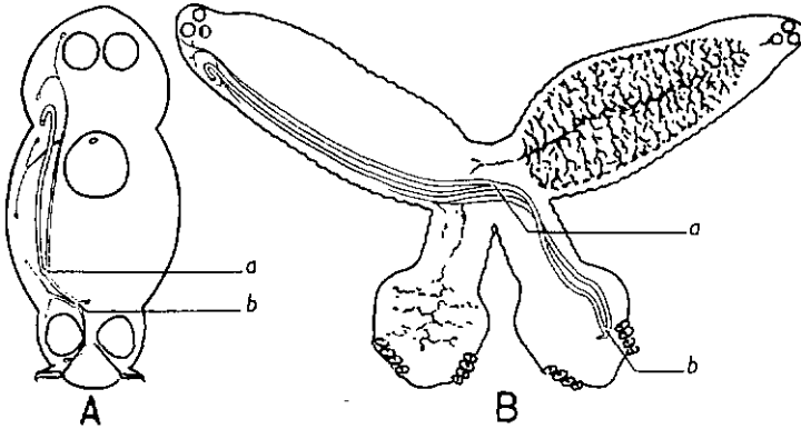
Fig. 25. Répartition des canaux excréteurs principaux : A : chez l'oncomiracidium ; B : chez l'adulte ; a et b : voir le texte.
