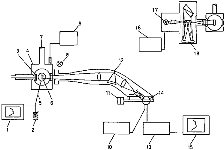
Fig. 11. Schéma de mesures des spectres d'émission d'un cristal irradié par une source \beta de Sr^{90} (40 mCi) ou une source de lumière monochromatique (illustration dans le coin supérieur droit).
