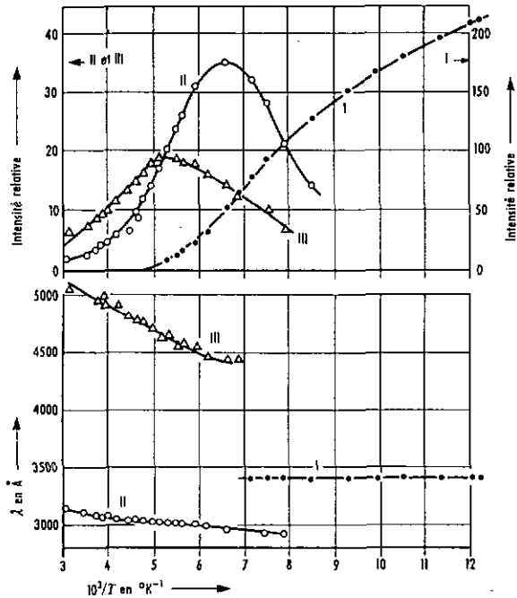
Fig. 17. Evolution avec la température du spectre d'émission d'un cristal purifié (série G5); seule la bande correspondant à \gamma_3 subsiste (I). La bande peu intense située entre 4500 et 5000 Å qui semble lui être associée est notée III. L'émission à 3000 Å également faible (II) est d'origine non identifiée.
