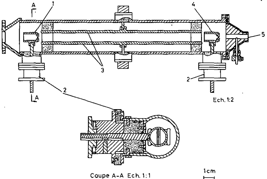
Fig. 8. Coupe schématique du déflecteur électrostatique.
