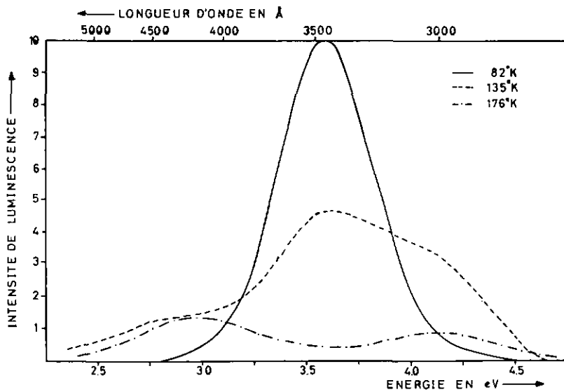
Fig. 14. Spectres d'émission corrigés d'un cristal de CsI (série B N° 3) irradié par une source \beta ( \text{Sr}^{90} ) et mesurés à 3 températures différentes. Le maximum à 3,6 eV (3450 Å) aux basses températures et qui disparaît au-dessus de 200° K correspond à la composante froide \gamma_2 . La bande d'émission voisine de 2,9 eV (4300 Å) constitue la composante chaude \gamma_1 .
