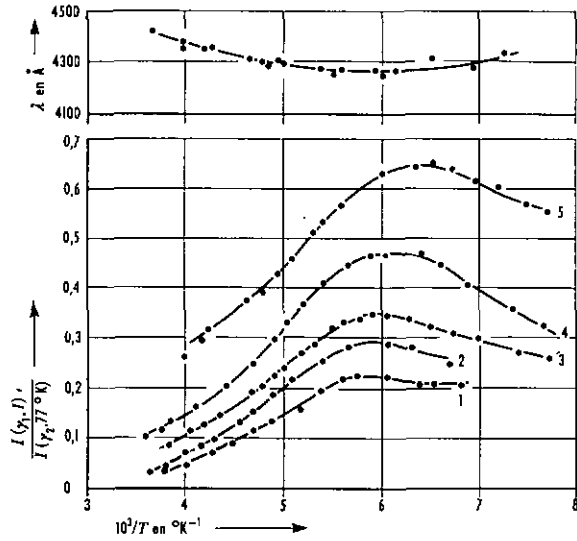
Fig. 16. Variation du rapport d'intensité I_{\gamma_1}(T) / I_{\gamma_1}(77^\circ \text{K}) pour cinq cristaux purifiés par fonte zonale (série B). La concentration en ions divalents varie de 30 à 300 ppm respectivement pour les cristaux notés de 1 à 5.
