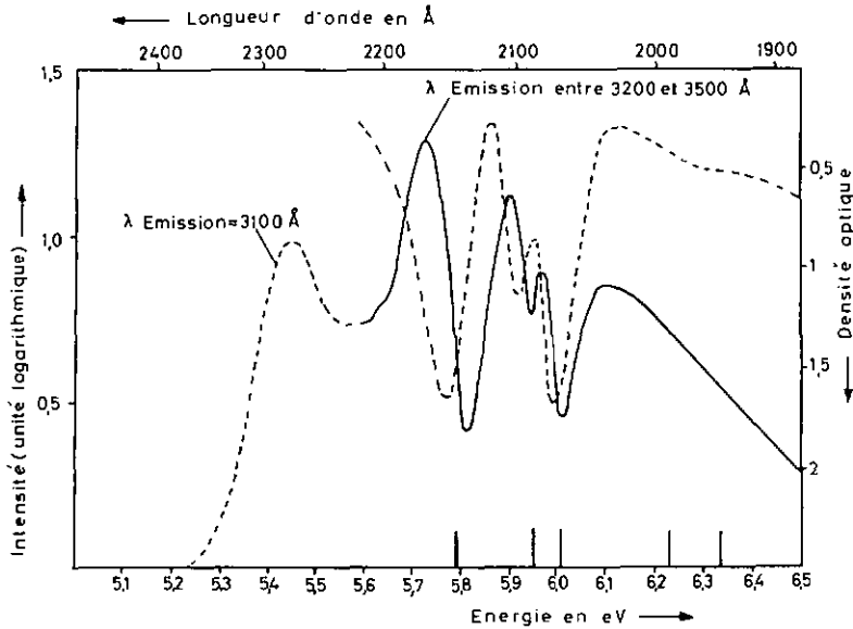
Fig. 19. Spectre d'excitation UV à 77° K montrant pour la composante \gamma_2 l'existence des maxima à 5,96; 5,90 et 5,73 eV correspondant aux pics d'excitons mesurés en absorption avec un décalage analogue à celui observé pour KI et NaI. La courbe en pointillés est le spectre d'absorption (ÉBY, TEGARDEN et DUTTON (1959)) renversé. Les positions des maxima d'absorption d'après FISCHER et HILSCH (1959) sont également indiquées.
