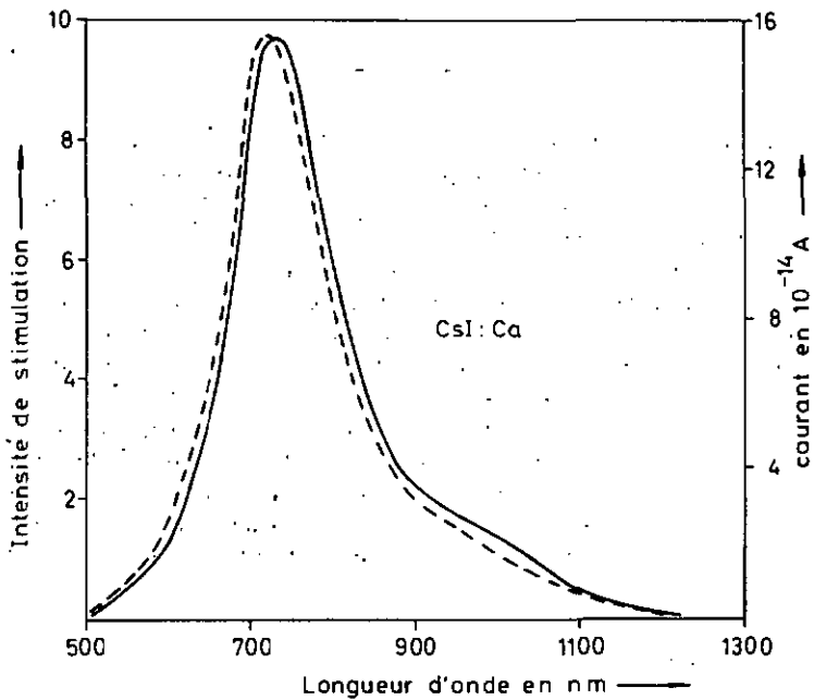
Fig. 34. Enregistrement simultané de photocourant et de stimulation IR dans CsI : Ca, après irradiation \beta à 57° K. La tension appliquée aux électrodes est de 270 V. ——— luminescence stimulée - - - - - photocourant.
