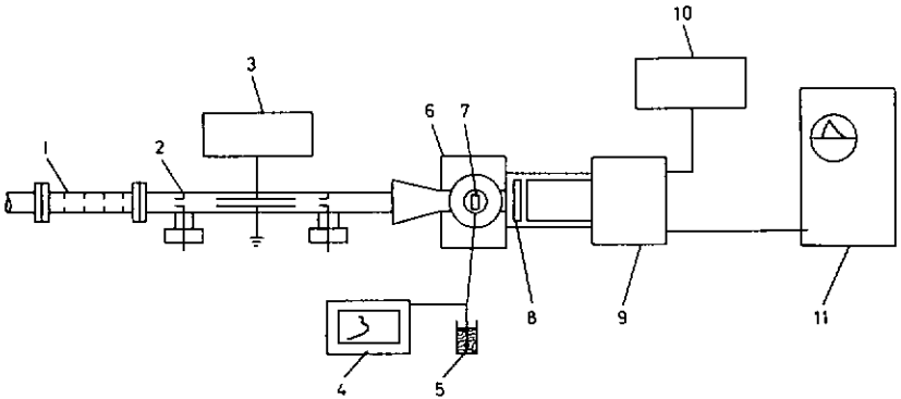
Fig. 13. Schéma de mesures des scintillations lumineuses par irradiation pulsée de protons de 1 MeV.
