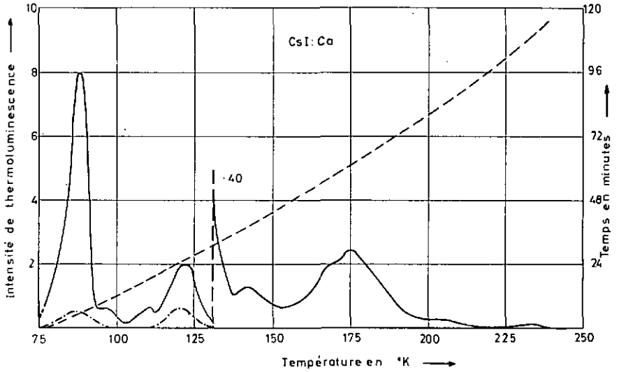
Fig. 26. Thermoluminescence de CsI : Ca après irradiation \beta de 15 minutes à 77° K. La courbe en trait discontinu correspond à la mesure de la température. Il est également représenté dans la figure l'enregistrement de thermoluminescence effectué après une stimulation IR à 750 nm. Les enregistrements de thermoluminescence de CsI : Sr et CsI : Mn sont essentiellement identiques.
