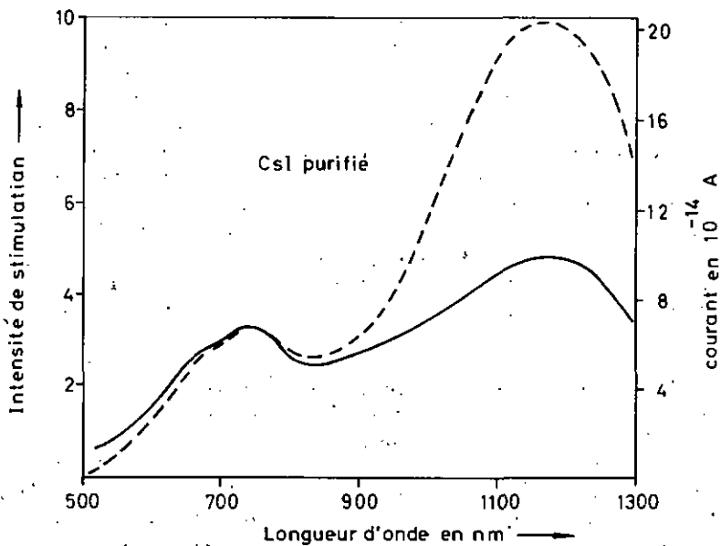
Fig. 35. Enregistrement simultané de photocourant et de stimulation IR dans CsI purifié (série G2) après irradiation \beta à 57° K. La tension appliquée aux électrodes est de 270 V. ——— luminescence stimulée - - - - - photocourant.
