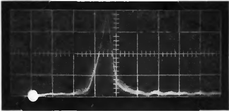
Fig. 10. Forme d'impulsion, recueillie à l'anode d'un PM 56 UVP ( R = 125 \Omega ), pour un scintillateur de Ne 102 soumis à une irradiation de protons pulsés de 1 MeV dans les conditions expérimentales décrites ci-dessus. 1 division = 20 ns.
