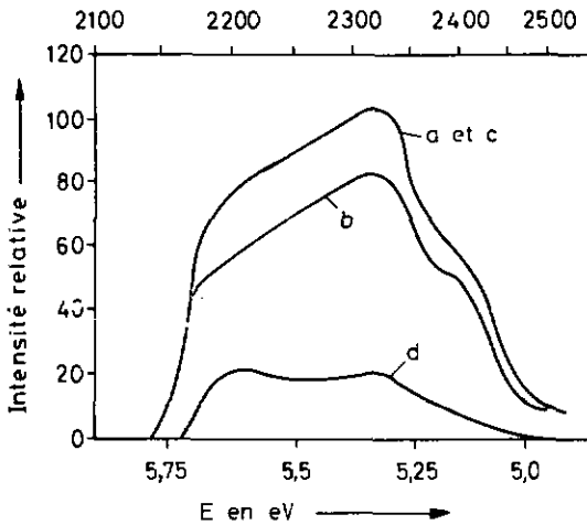
Fig. 23. Influence d'une irradiation \beta à 57° K sur le spectre d'excitation UV de \gamma , dans CsI: Ca.
