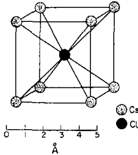
Fig. 1. Structure des halogénures d'alcalins du type CsCl.
