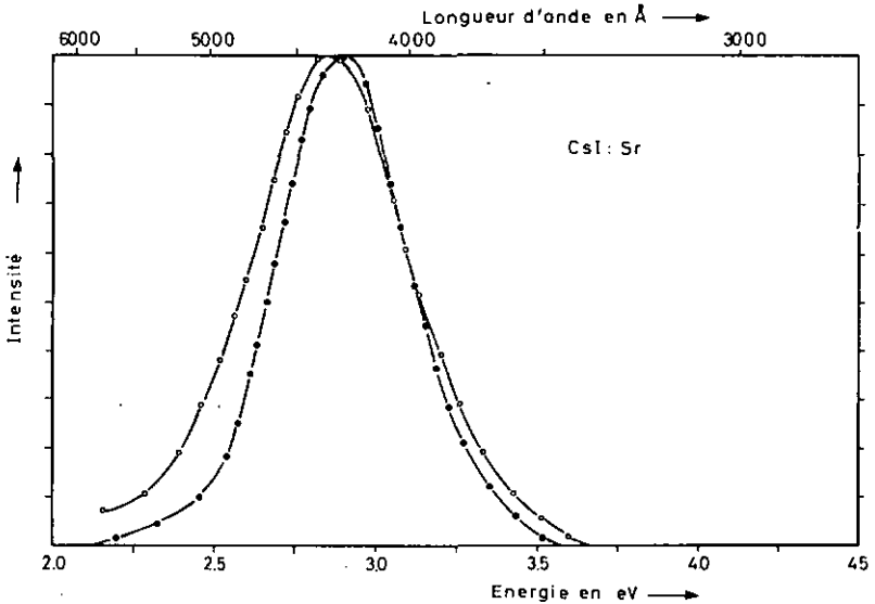
Fig. 27. Forme des bandes d'émission observées au maximum d'intensité des deux premiers pics thermoluminescents des cristaux dotés (exemple CsI : Sr). ● 86° K émission à 2,9 eV (4280 Å). ○ 122° K émission à 2,85 eV (4350 Å).
