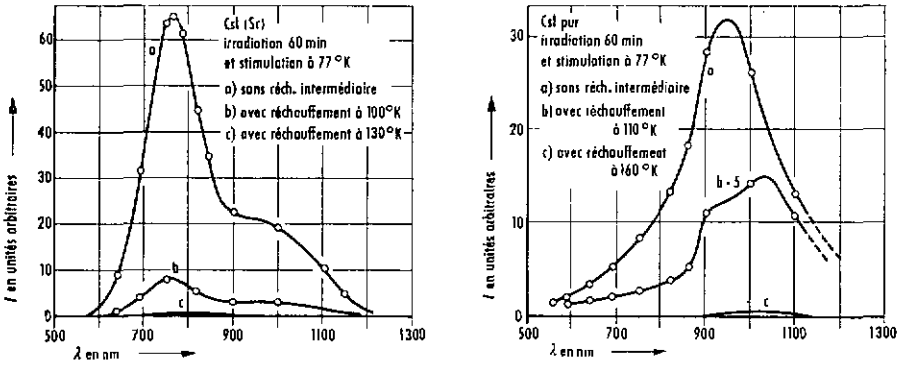
Fig. 30. Stimulation IR de cristaux préalablement irradiés par les \beta à 77° K. La bande de stimulation à 750 nm présente dans les cristaux dotés est attribuée à la formation de centre Z_1 (électron piégé sur un complexe ion divalent — lacune cationique). La bande non résolue vers 950 nm observée dans les cristaux dotés et dans les cristaux purifiés avec une intensité semblable est probablement liée à la présence d'impuretés inconnues. La forte atténuation des bandes de stimulation après réchauffement intermédiaire à 110° K peut s'expliquer par la recombinaison de centres V_K thermiquement instables vers 87° K sur ces pièges à électrons.
