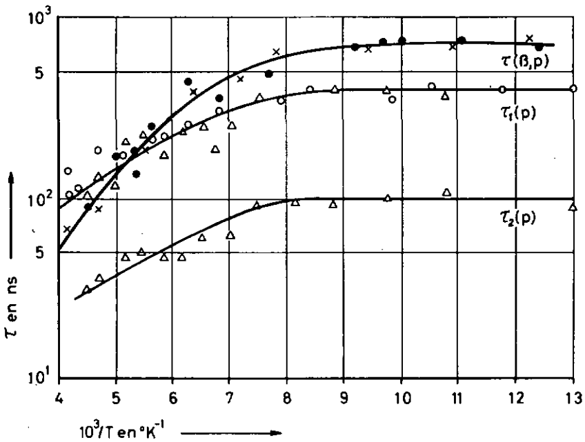
Fig. 25. Temps de déclin en fonction de la température pour irradiation par protons (O, Δ) (doublet, série G2) et pour irradiation β (●) et protons (x) (bande unique série G5).
