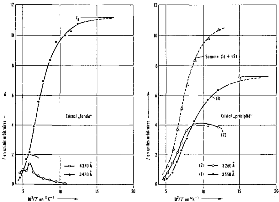
Fig. 15. Variation avec la température de l'intensité émise dans la composante \gamma_2 par excitation \beta ( \text{Sr}^{90} ). Pour le cristal «fendu» le doublet n'apparaît pas et l'émission a lieu à 3470 Å. Le rendement est identique à la somme des deux pics observés pour un cristal tiré de la solution aqueuse.
