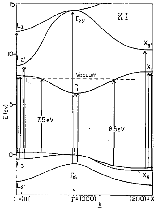
Fig. 4. Schéma de bandes d'énergies du KI le long des axes [100] et [111] d'après PHILLIPS (1964 et 1966).
