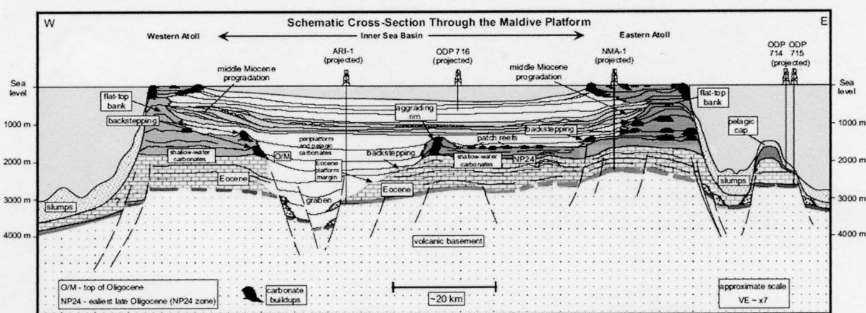
Figure 4. Structure des récifs des Maldives, d'après Belopolsky et Droxler (2004), simplifiée.
