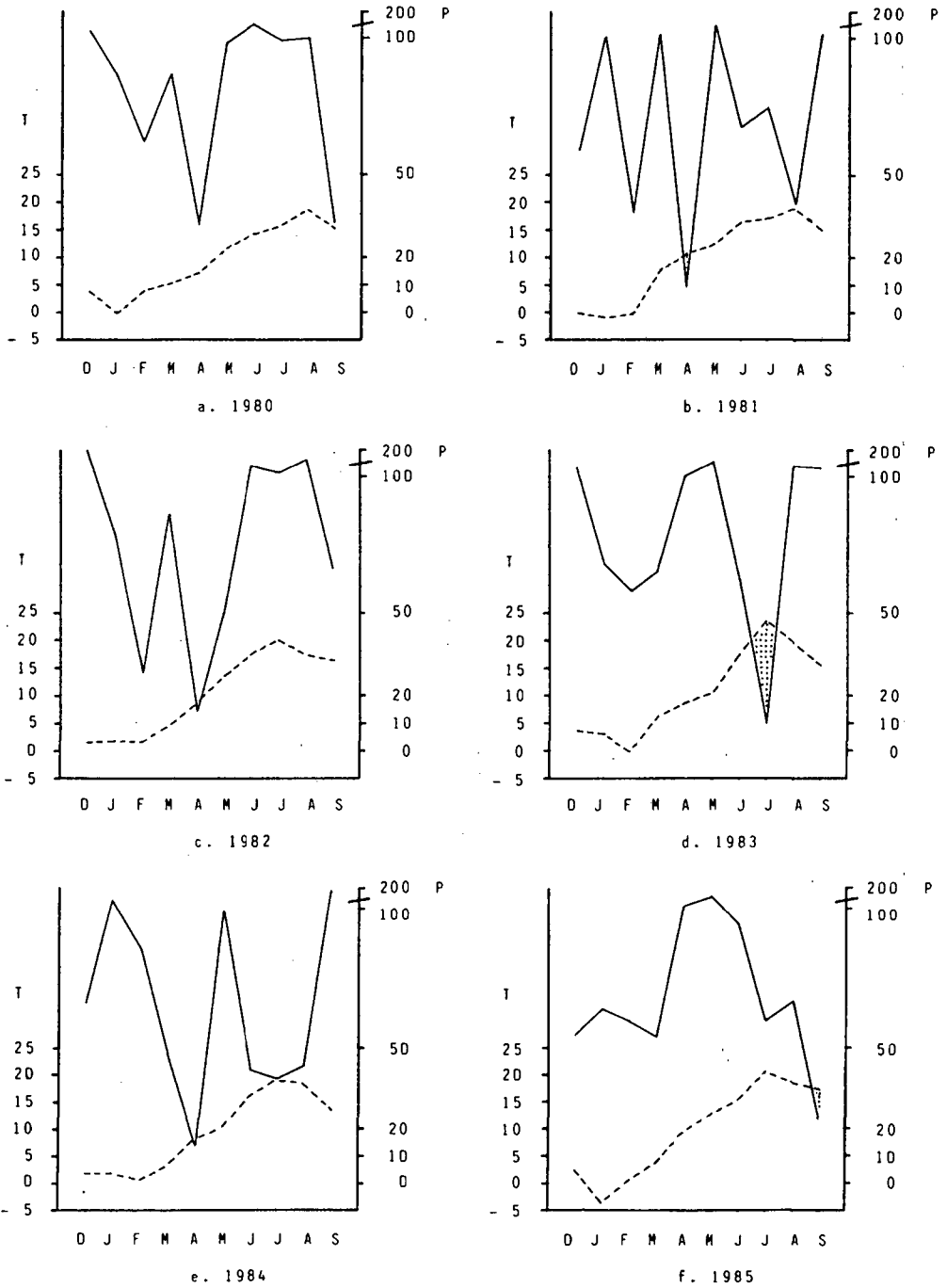
Fig. 6.17.a-f. Diagrammes ombrothermiques de Neuchâtel, de 1980 à 1985, entre saisons de chasse (de décembre (an préc.) à septembre). P, en continu: pluviosité (mm). T, en traitillé: température (°C). Sécheresse (pointillés) lorsque P_{\text{mm}} < 2 T_{\text{°C}} (selon GAUSSEN).
