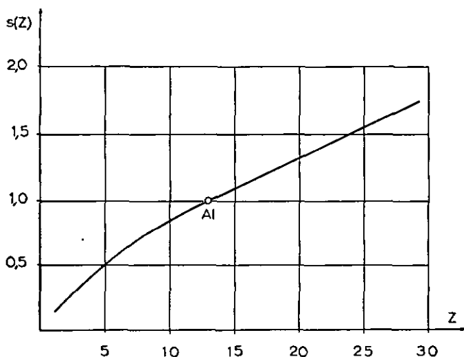
Fig. 4. Pouvoir d'arrêt atomique par rapport à l'Al en fonction du numéro atomique Z .
