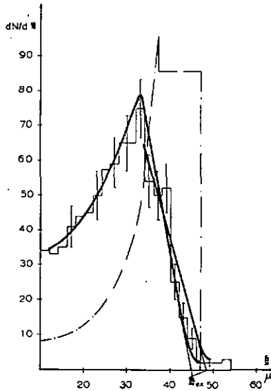
Fig. 6. Distribution des parcours des protons dans l'émulsion Ilford C 2 . N t =818 traces ( \theta \geq 20^\circ ) ; largeur de classe 2 \mu ; 44,8 < \xi_{ex} < 48,4 \mu ; \xi_{ex} = (46,6 \pm 1,8) \mu . La courbe en traits-points donne la répartition prévue calculée.
