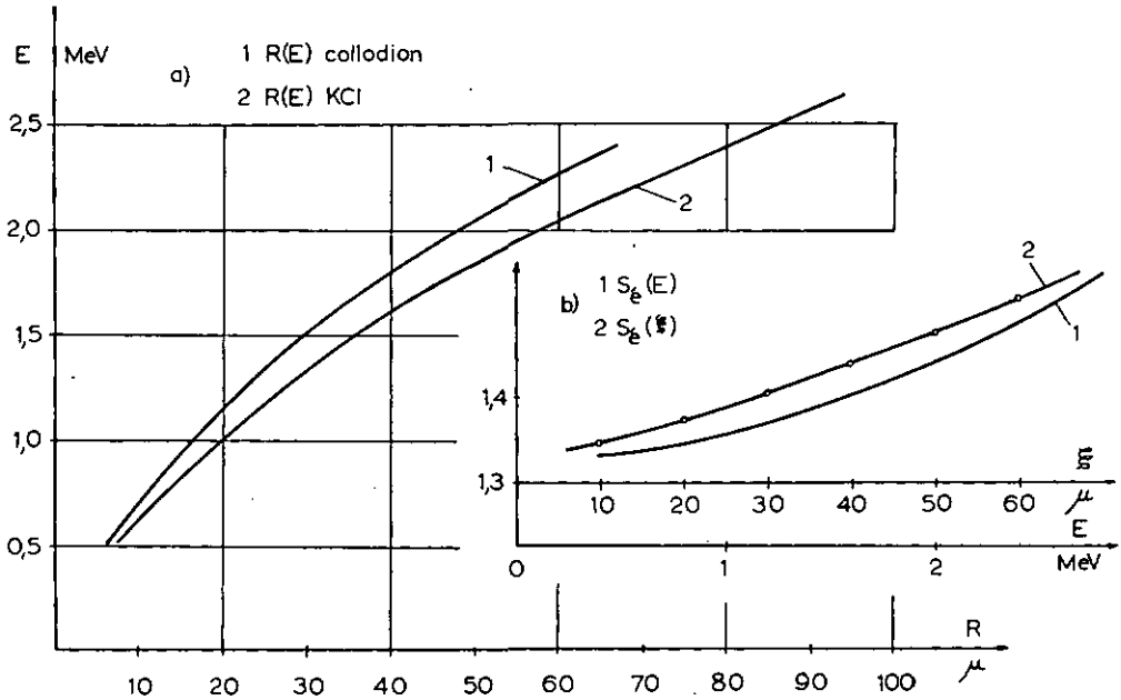
Fig. 5a. Courbes parcours-énergie : 1) collodion, 2) KCl.
