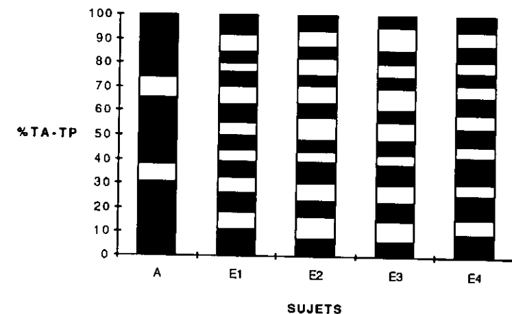
Figure 1 : Le rythme des sujets basé sur la répartition temporelle du temps d'articulation (TA) et du temps de pause (TP) en pourcentages. Chaque zone noire représente le temps d'articulation (6 mesures en moyenne) et chaque zone blanche représente le temps de pause (6 mesures en moyenne).
