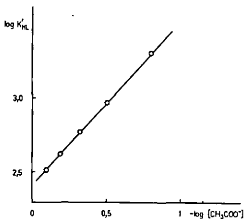
Fig. 3. Variation de K'_{\text{ML}} en fonction de la concentration en \text{CH}_3\text{COO}^- pH = 5,5; [\text{NaCH}_3\text{COO}] + [\text{NaClO}_4] = 0,8\text{M} , [\text{phen}] = 8 \cdot 10^{-5}
