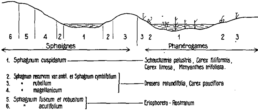
FIG. 7. Coupe d'un kolk.
