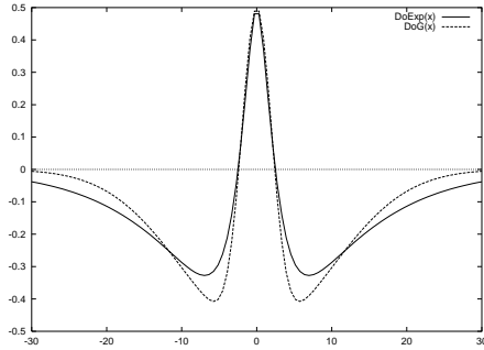
Fig. 3. \mathcal{D}\circ\mathcal{E}xp versus \mathcal{D}\circ\mathcal{G} .
