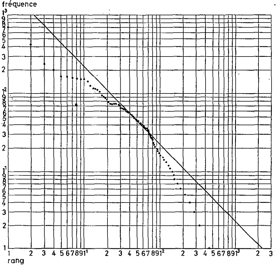
Courbe bilogarithmique de la distribution rang-fréquence
