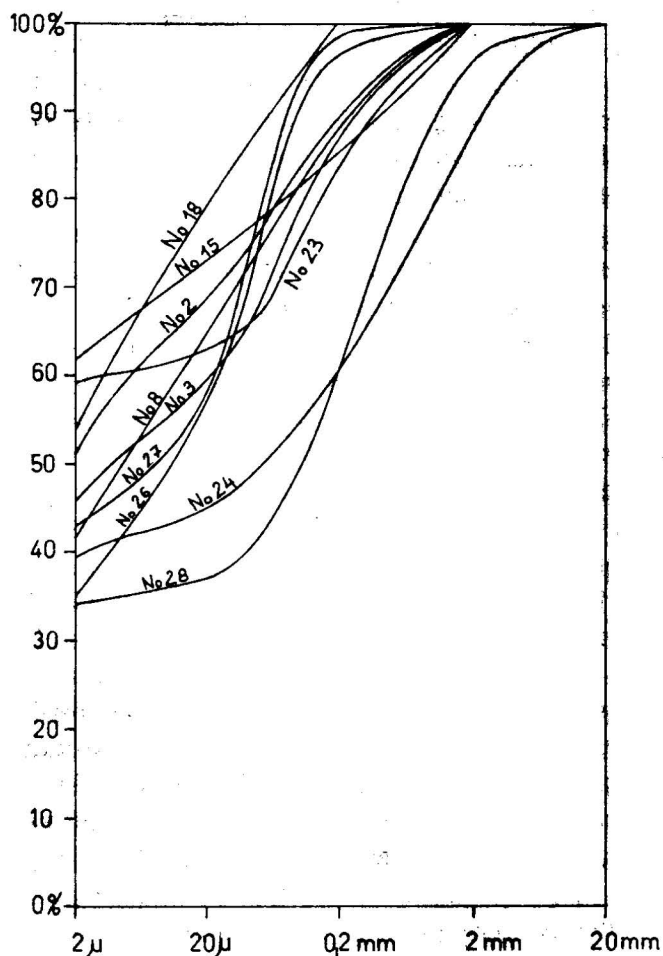
Fig. 4. Courbes cumulatives du résidu insoluble en HCl de quelques échantillons
