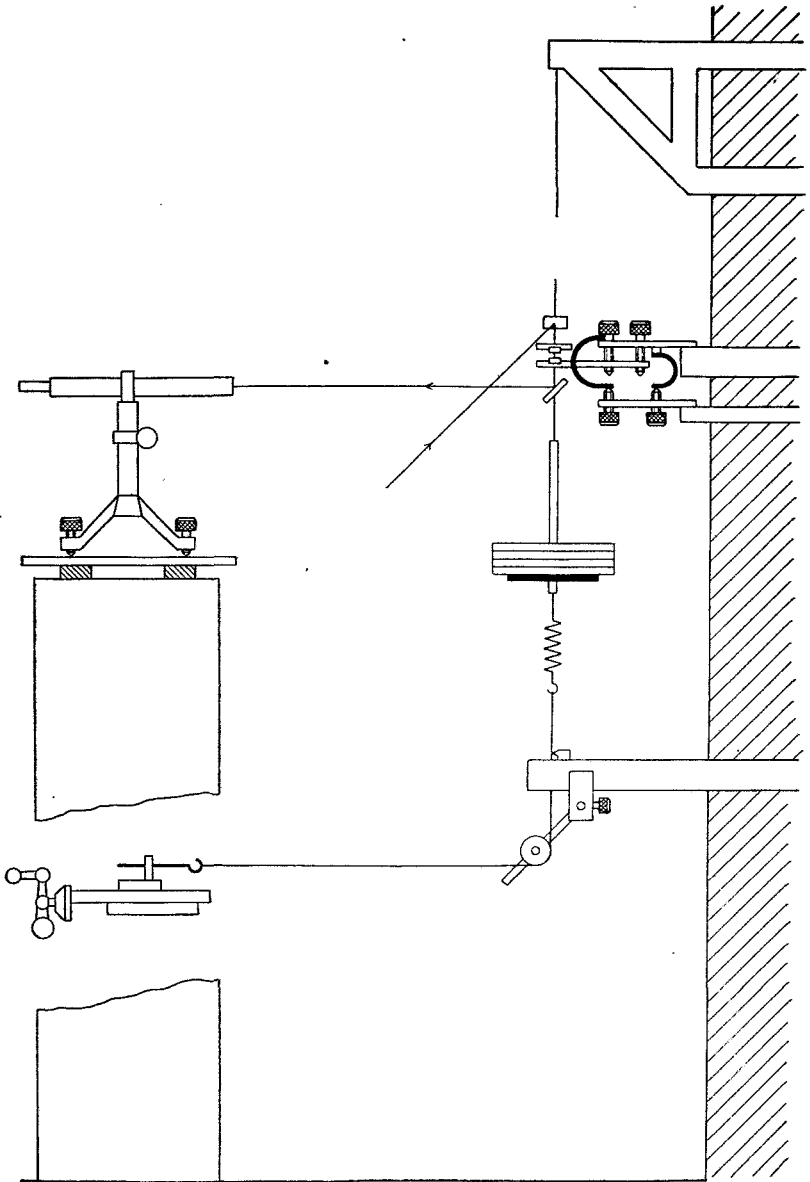
Fig. 1. Schéma de l'appareil.
