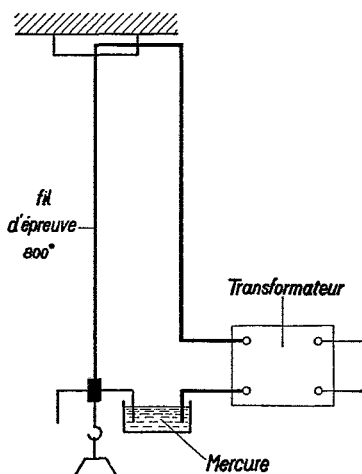
Fig. 6. Recuit des fils de cuivre à l'aide du courant électrique.
