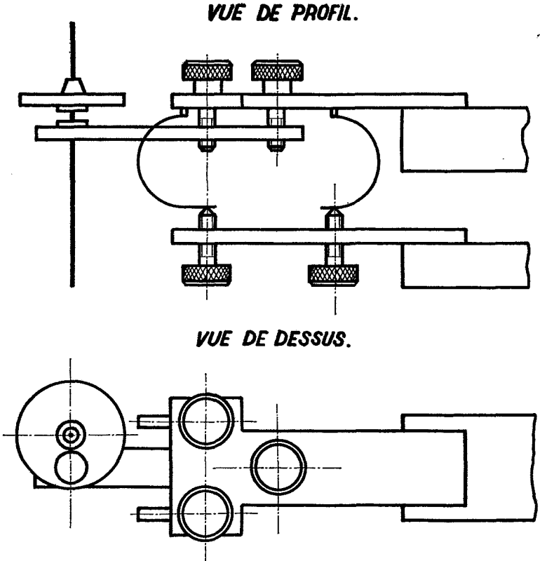
Fig. 3. Schéma de l'interféromètre et de son réglage.
