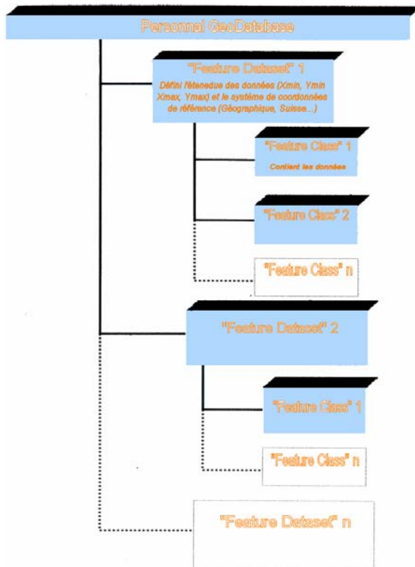
Fig 2 Relation entre « Personal Geodatabase », « Feature Dataset » et « Feature Class ». (modifié d'après exercice Bouzelboudjen, 2005)
