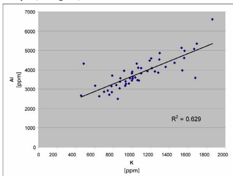
Fig 8.5 Graphique d'Al en fonction de K démontrant l'analogie du comportement de ces éléments.
