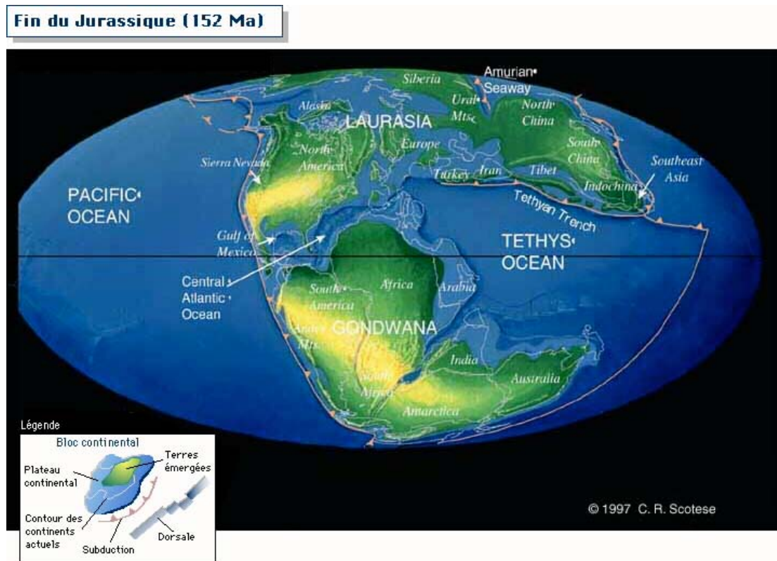
Fig 2.3 Situation paléogéographique à la fin du Jurassique. (d'après Scotese, site internet)
