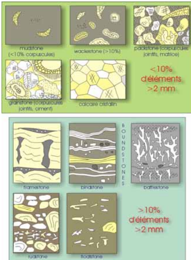
Fig 5.2 Classification de Dunham (1962), élargie par Embry & Klován (1971).
