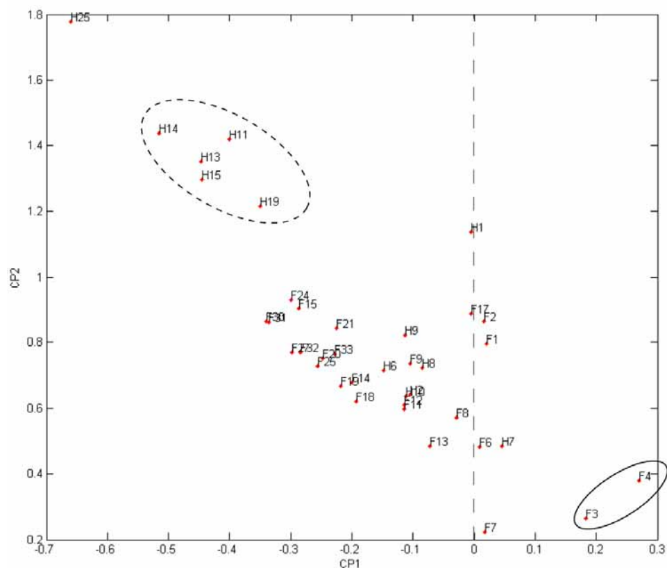
Fig 8.21 Echantillons exprimés selon CP1 et CP2.
