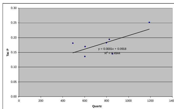
Fig 10.6 Comparaison entre les taux d'accumulation du phosphore et du quartz sur les échantillons autour de la limite KT. Une droite de régression linéaire a été calculée.
