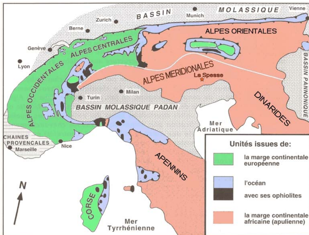
Fig 2.4 Schéma structural des Alpes, montrant la répartition des unités d'origine européenne, océanique (liguro-piémontaise) et apulo-africaine. (modifié d'après Lemoine et al., 2000)
