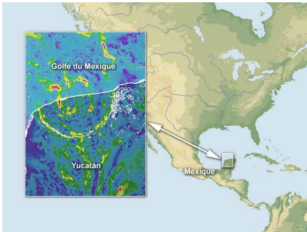
Fig 1.2 Localisation du Cratère de Chicxulub.
