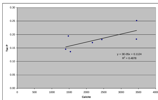
Fig 10.4 Comparaison entre les taux d'accumulation du phosphore et de la calcite sur les échantillons autour de la limite KT. Une droite de régression linéaire a été calculée.
