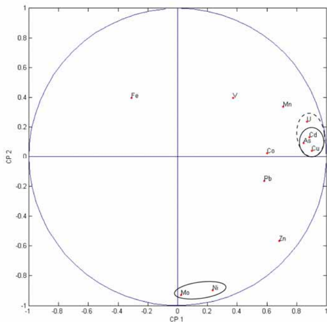
Fig 8.18 Cercle de corrélation selon CP1 et CP2.
