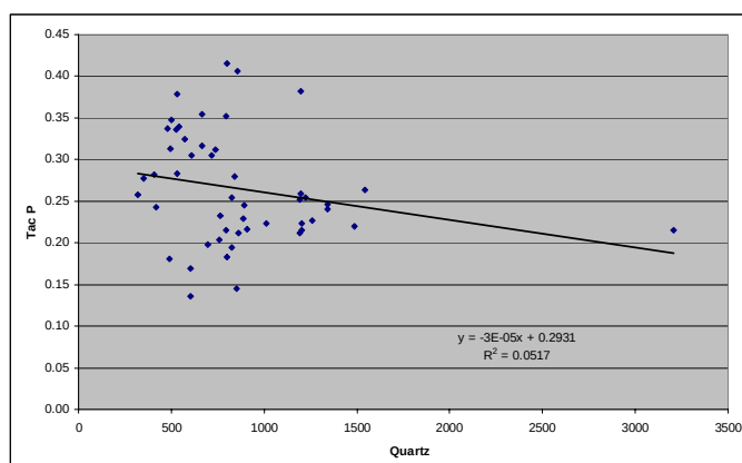
Fig 10.5 Comparaison entre les taux d'accumulation du phosphore et du quartz sur les échantillons F33 à H36 de la coupe de La Spesse. Une droite de régression linéaire a été calculée.
