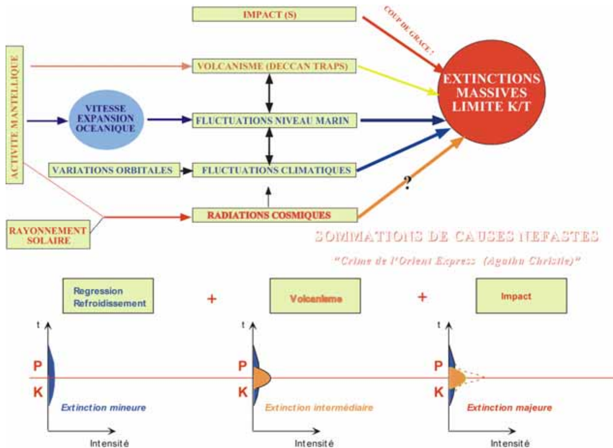
Fig 1.5 Schéma explicatif de la conjonction de causes et de la superposition de facteurs néfastes lors de l'extinction en masse de la limite KT. (modifié selon Lethiers, 1998 ; Erwin, 1993 ; Hallam et Wignall, 1998 par T. Adatte, 2003)
