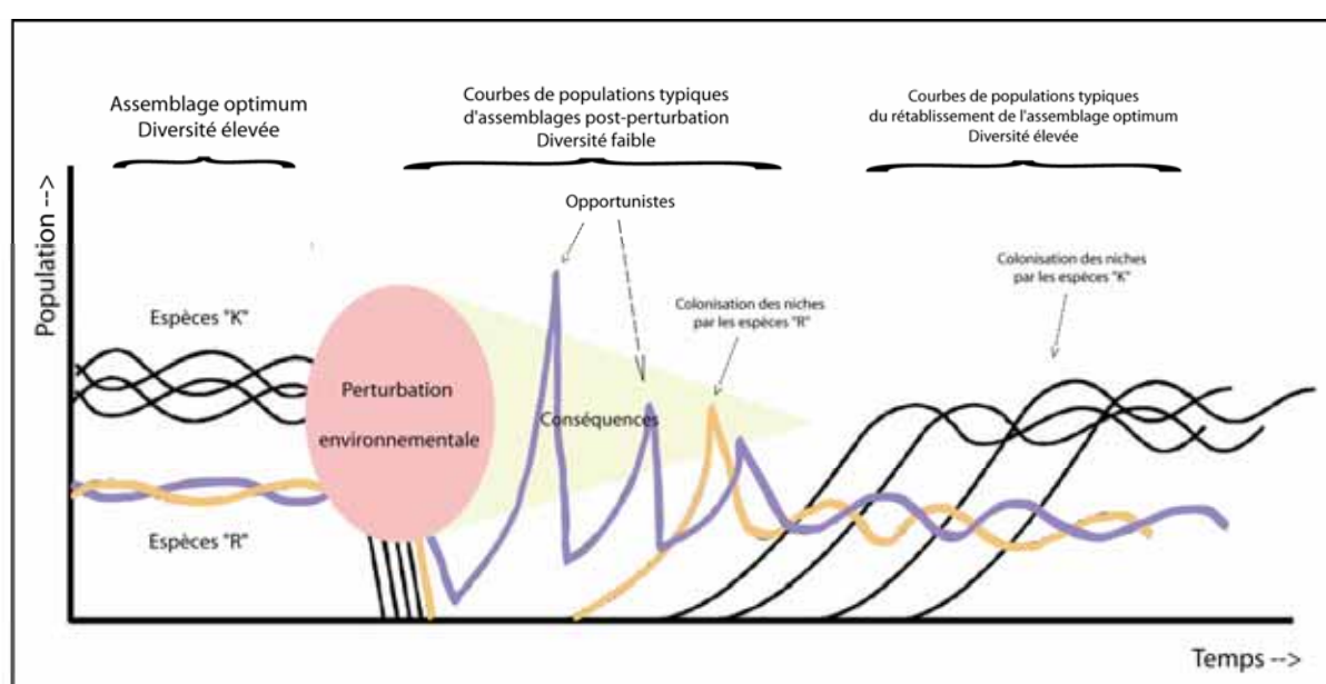
Fig 6.1 Modèle illustrant la succession écologique après une perturbation environnementale majeure. (modifié d'après Keller et Pardo, 2004)
