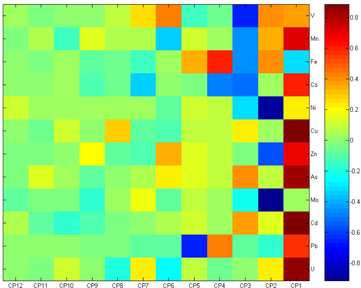
Fig 8.16 Figure illustrant les différentes composantes principales et leur corrélation avec les éléments étudiés selon un code couleur.
