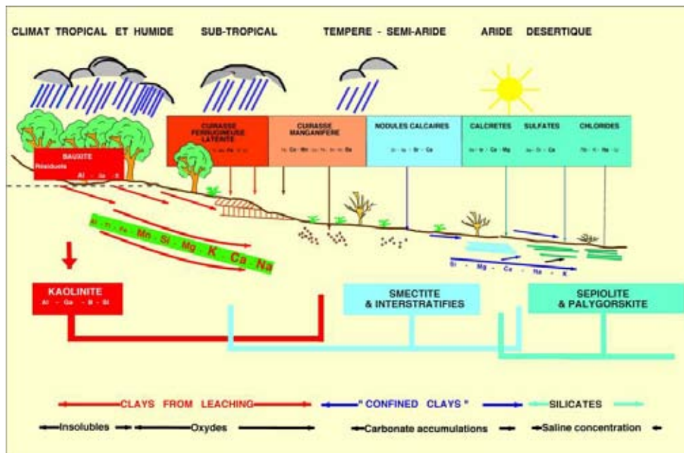
Fig 7.4 Altération superficielle et néoformation des minéraux argileux en fonction des différentes zones climatiques. (Adate 2005, modifié d'après Tardy 1981)
