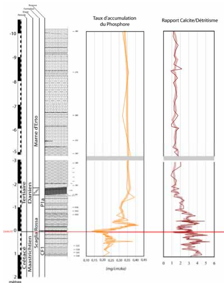
Fig 10.2 Comparaison entre les taux d'accumulation du phosphore et le rapport calcite/détritisme dans la coupe de La Spesse.
