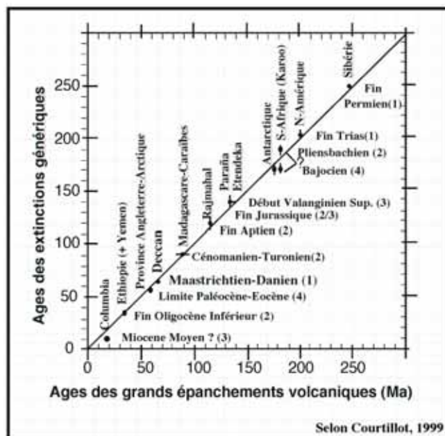
Fig 1.4 Relation entre les périodes de volcanisme intense et les extinctions en masse.
