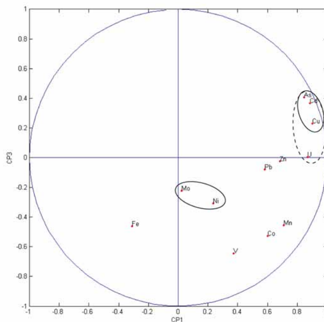
Fig 8.19 Cercle de corrélation selon CP1 et CP3.
