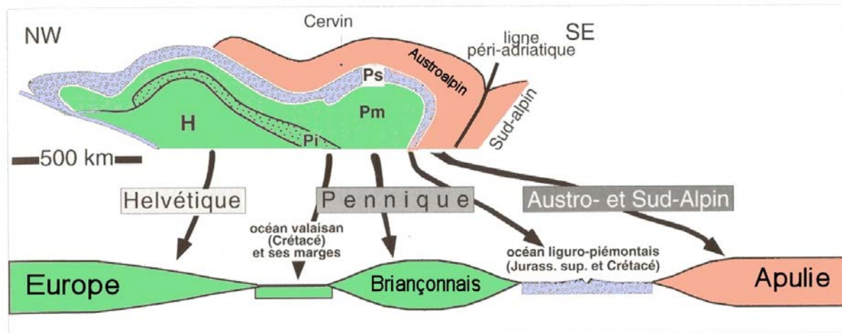
Fig 2.5 Schéma des subdivisions majeures des Alpes. En haut : Superposition actuelle des unités tectoniques. En bas : Reconstitution au Jurassique. (modifié d'après Lemoine et al., 2000)
