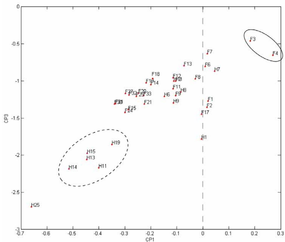
Fig 8.22 Echantillons exprimés selon CP1 et CP3.
