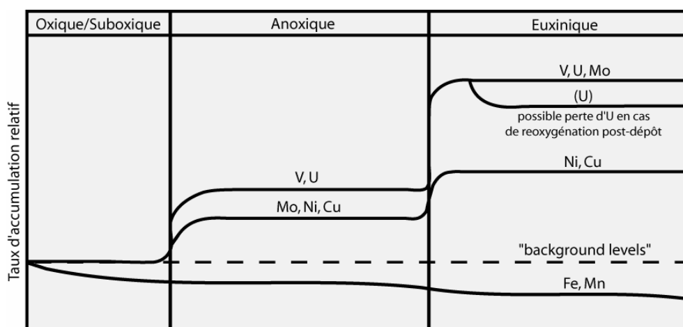
Fig 8.3 Comportement de Ni, Cu, Mo, V et U en fonction de conditions redox de l'environnement de dépôt. (modifié d'après Algeo et Maynard, 2004)
