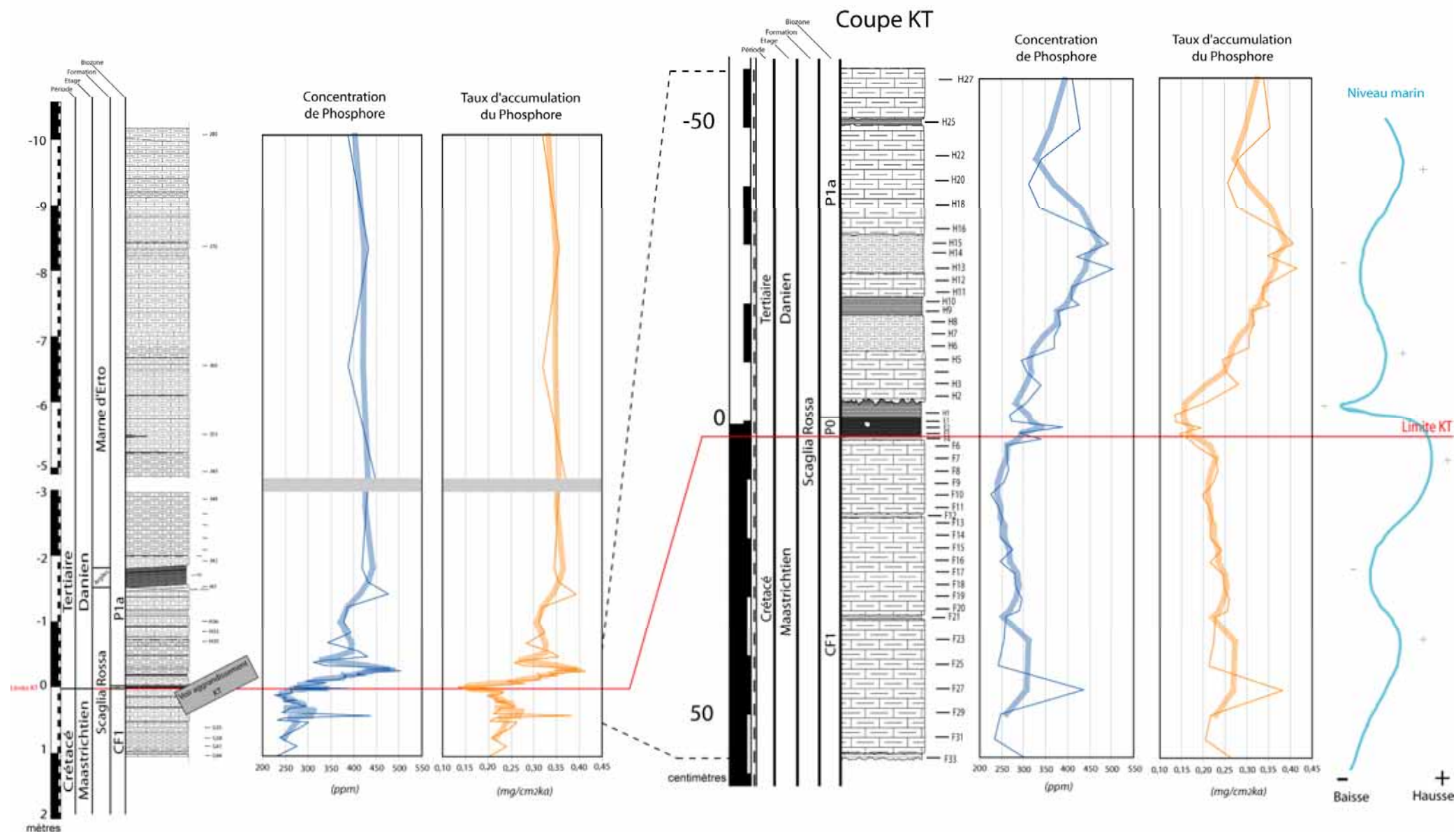
Fig 10.1 Concentration et taux d'accumulation du phosphore dans la coupe de La Spesse ainsi que la courbe du niveau marin obtenu au chapitre 7 (Minéralogie).
