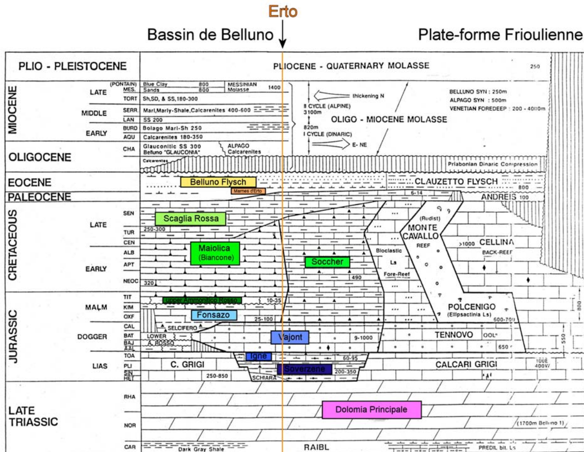
Fig 2.10 Stratigraphie généralisée de la marge continentale apulo-africaine. (modifiée d'après Zappaterra, 1990)
