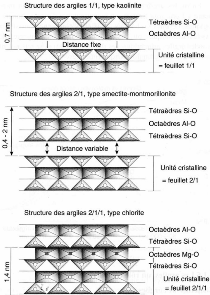
Fig 7.3 Structure minéralogique des argiles. (d'après Gobat et al., 2003)
