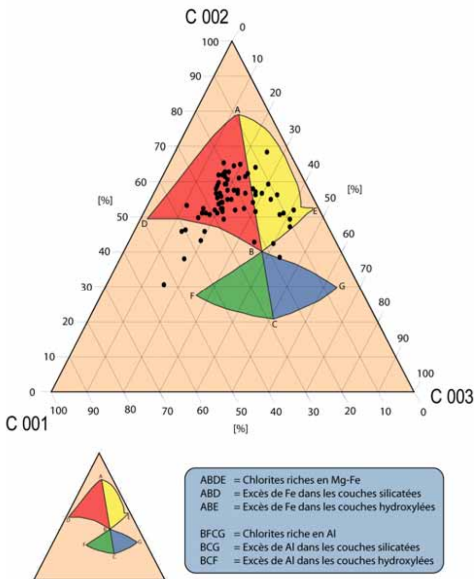
Fig 7.6 Diagramme ternaire de la chlorite pour la fraction 2-16 \mu m
