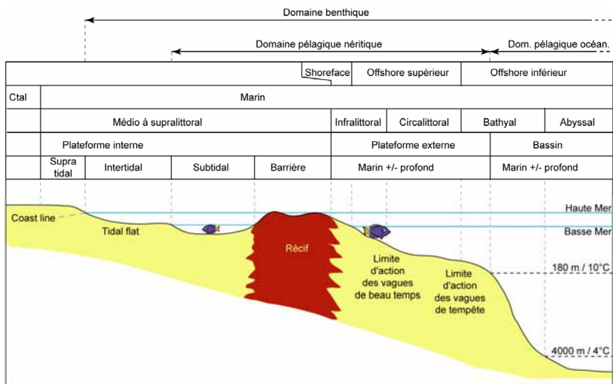
Fig 5.5 Schéma montrant la répartition des différents environnements dans une plateforme carbonatée possédant une barrière récifale.
