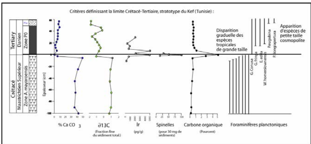
Fig 1.6 Critères définissant le GSSP de la limite KT à Kef, Tunisie. (Adatte, 2003)
