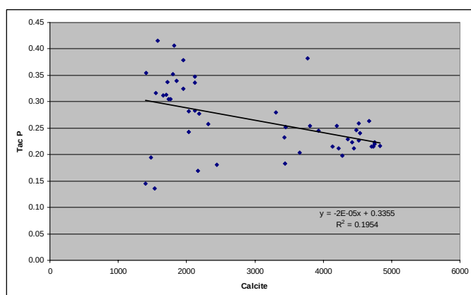
Fig 10.3 Comparaison entre les taux d'accumulation du phosphore et de la calcite sur les échantillons F33 à H36 de la coupe de La Spesse. Une droite de régression linéaire a été calculée.
