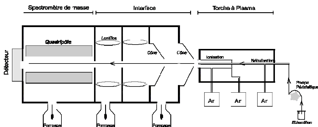
Fig 8.1 Schéma instrumental de l'ICP-MS.
