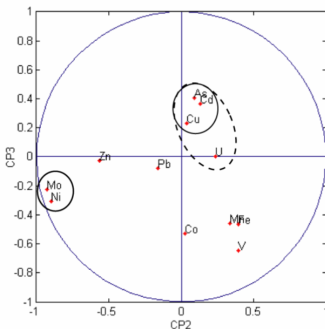
Fig 8.20 Cercle de corrélation selon CP2 et CP3.
