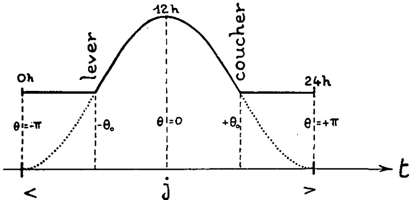
Fig. 4. — Variation journalière de l'apport d'énergie solaire.
