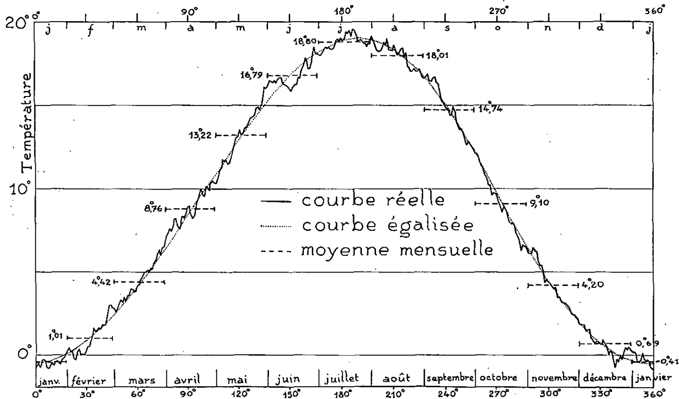
Fig. 1. — Courbe de la variation annuelle de la température journalière, tracée jour par jour (moyenne 1864-1943).
