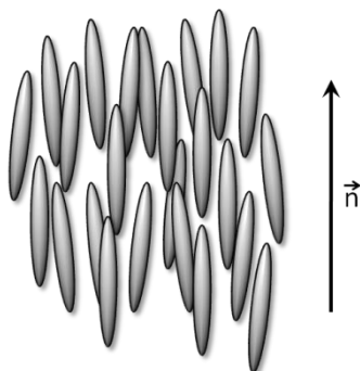
Figure 3. Modèle structurel de la phase nématique.
