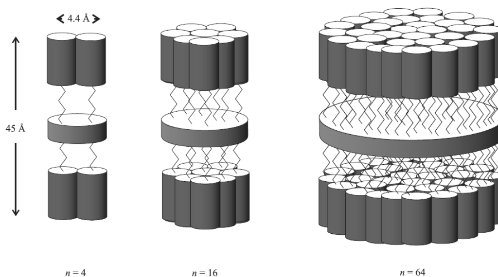
Figure 15. Modèle d'organisation dans la phase SmA pour les générations 1, 3 et 5 du dendrimer PPI fonctionnalisé par le mésogène décylloxycyanobiphényle. [95]
