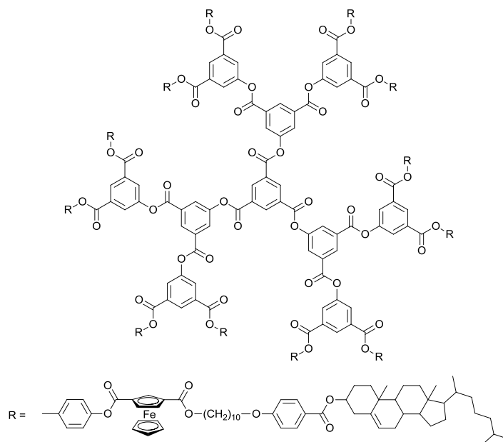
Figure 23. Métallomésogène à base de ferrocène décrit par Deschenaux.
