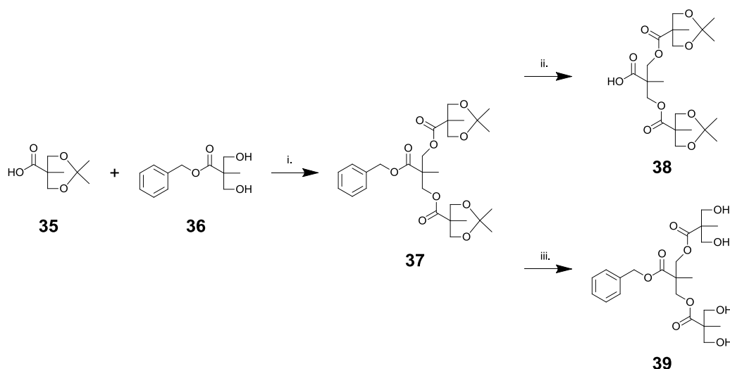
Schéma 16. i. DCC, DPTS, \text{CH}_2\text{Cl}_2 sec, t.a. 1 nuit, 36 % ; ii. \text{H}_2 , Pd/C, AcOEt, t.a. 1 nuit, 99 % ; iii. Dowex \text{H}^+ , MeOH, t.a. 3h, 100 %.
