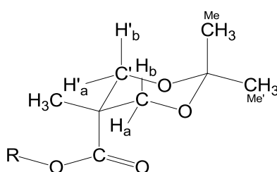
Figure 51. Conformation chaise du cycle à six atomes du dendrimer polyester.
