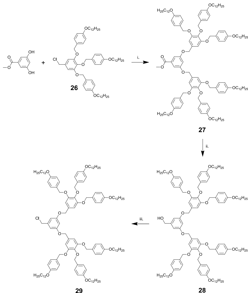
Schéma 12. i. \text{K}_2\text{CO}_3 , DMF, THF, 1 nuit \Delta , 75 % ; ii. \text{LiAlH}_4 , THF sec, t.a. 2h, 84 % ; iii. DTBP, \text{SOCl}_2 , \text{CH}_2\text{Cl}_2 sec, t.a. 45 min, 62%.
