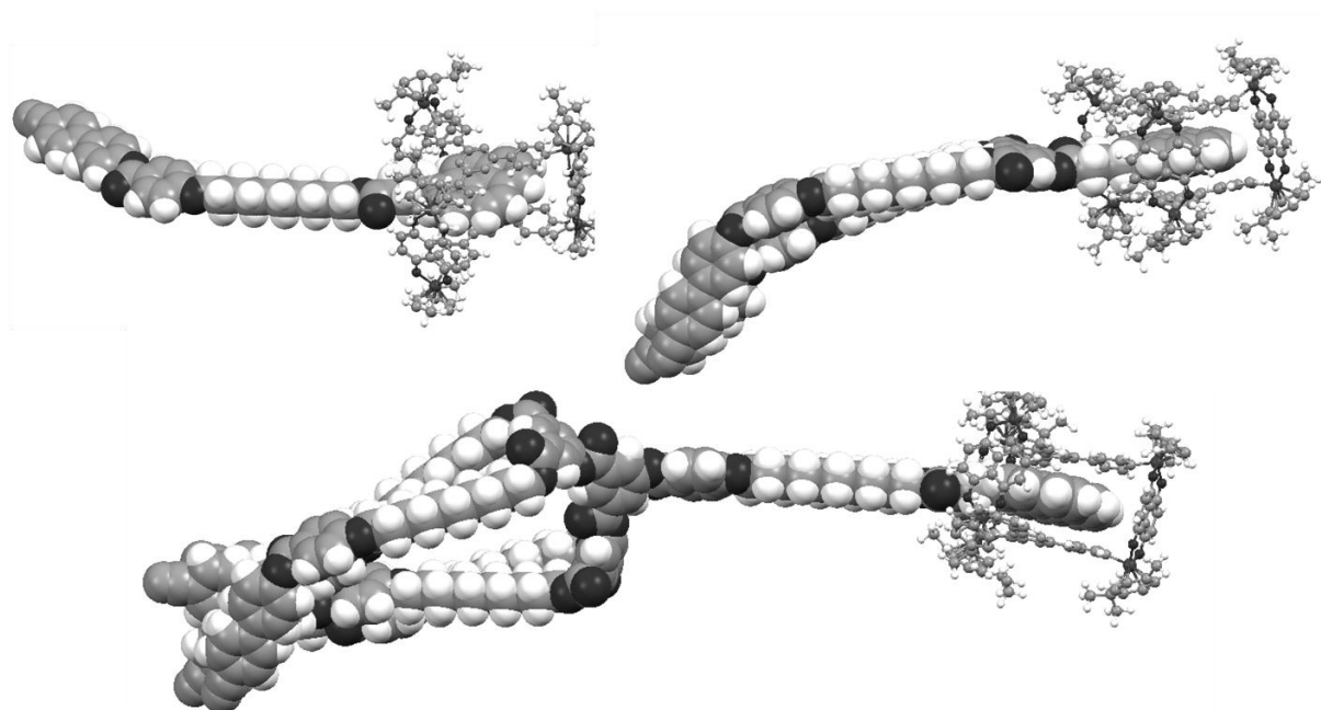
Figure 98. Simulation Hyperchem des systèmes host-guest 97 (en haut à gauche), 98 (en haut à droite) et 99 (en bas). Les contre-ions ont été omis pour une meilleure clarté.
