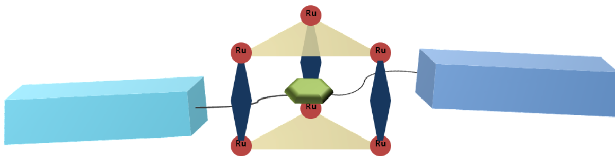
Figure 100. Encapsulation d'une unité poly-aromatique dans une cage prismatique. Les contre-ions sont omis.
