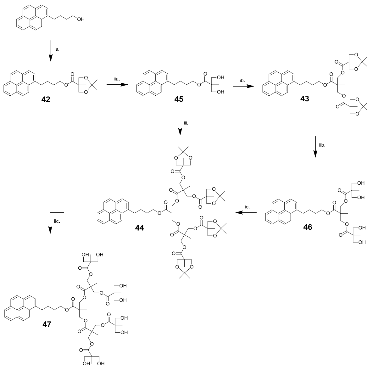
Schéma 19. i. Composé 35, DCC, DPTS, \text{CH}_2\text{Cl}_2 sec, t.a. 1 nuit ; a. 89 % ; b. 48 % ; c. 28 % ; ii. Dowex \text{H}^+ , MeOH, t.a. 3h ; a. 91 % ; b. 100 % ; c. 93 % ; iii. Composé 41, DCC, DPTS, \text{CH}_2\text{Cl}_2 sec, t.a. 1 nuit 42%.
