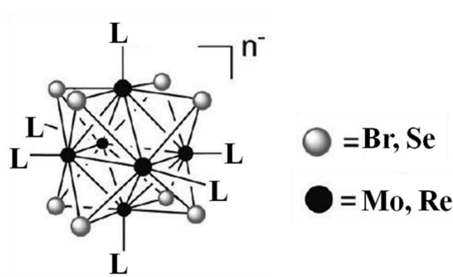
Figure 26. Clusters mésomorphes développés par Molard et Cordier.
