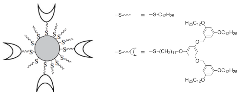
Figure 57. Représentation schématisée des nanoparticules d'or liquides-cristallines synthétisées par Donnio et Terazzi en 2007. [195]
