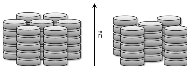
Figure 5. Modèles structuraux des phases colonnaires hexagonale (à gauche) et rectangulaire (à droite).
