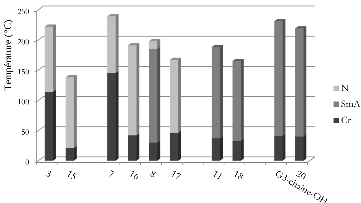
Figure 43. Variation de la température d'isotropisation en fonction de la génération du dendrimère et de la présence de l'unité pyrényle.
