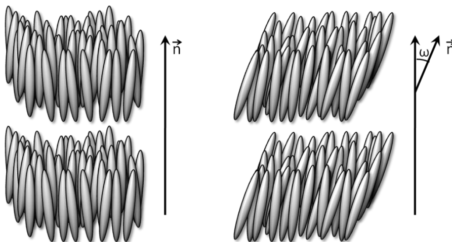
Figure 4. Modèles structurels des phases smectiques A (à gauche) et C (à droite).
