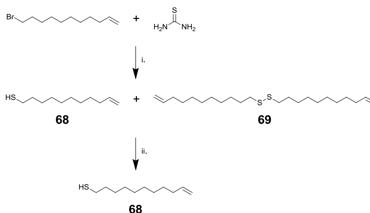
Schéma 30. i. EtOH, Δ 42h, NaOH 2N, Δ 42h ; ii. Zn, acide acétique, CH 2 Cl 2 , t.a. 4h ; rendement global 51%.
