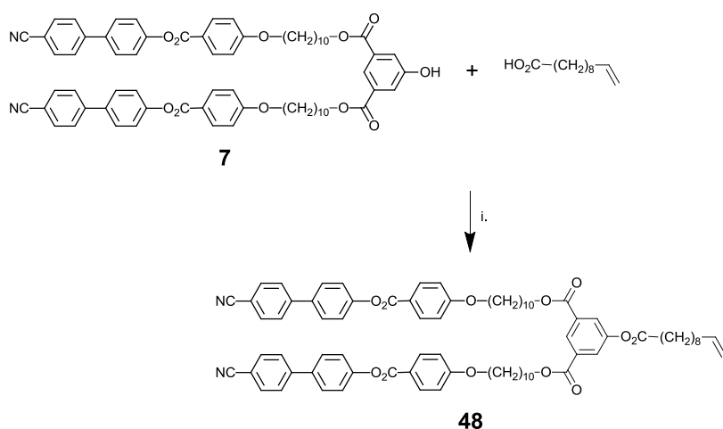
Schéma 21. i. DCC, DPTS, \text{CH}_2\text{Cl}_2 sec, t.a. 1 nuit, 75%.
