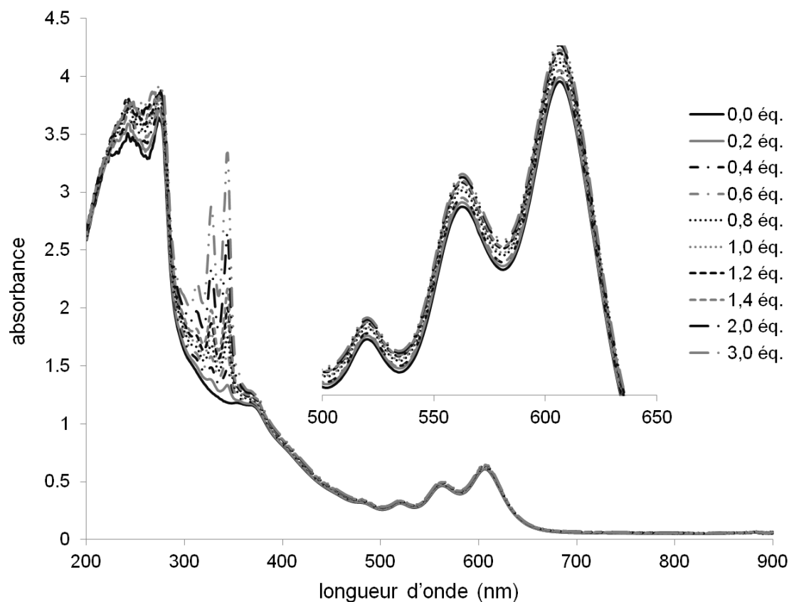
Figure 97. Spectres UV-Vis du dosage de la cage 94 (concentration de 10^{-4} \text{ mol}\cdot\text{L}^{-1} ) par le dendrimère fonctionnalisé 43 dans le dichlorométhane à 21°C.
