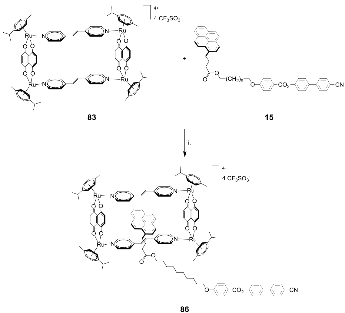
Schéma 39. i. \text{CH}_2\text{Cl}_2 , t.a. 1 jour, 100%.
