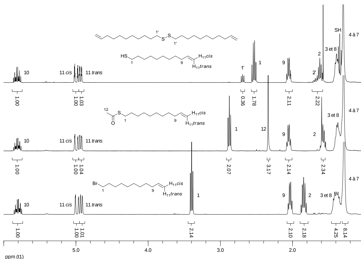
Figure 63. Spectres 1 H-RMN (400 MHz, CDCl 3 ) du 11-bromo-1-undécène (en bas), du composé 70 (au milieu) et du composé 68 et de son impureté 69 (en haut).
