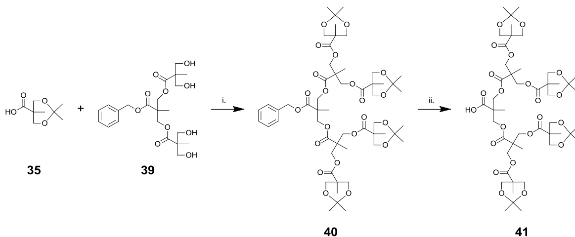
Schéma 17. i. DCC, DPTS, \text{CH}_2\text{Cl}_2 sec, t.a. 1 nuit, 63 % ; ii. \text{H}_2 , Pd/C, AcOEt, t.a. 1 nuit, 98 %.
