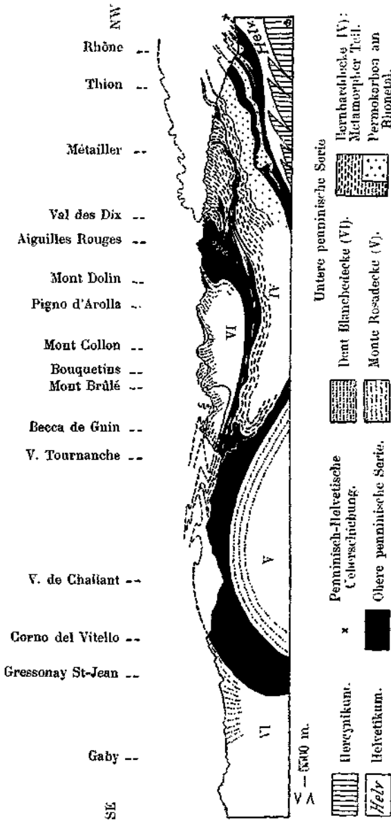
Fig. 2. Querschnitt durch die penninischen Alpen nach ARGAND, ergänzt nach den Aufnahmen des Verf. (1:500.000).
