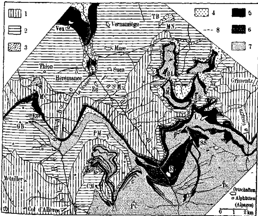
Fig. 1. Geologisches Uebersichtskärtchen (übernommen aus [7?]).
