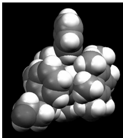
[C_6H_6\text{-}c\text{-}4]^+
