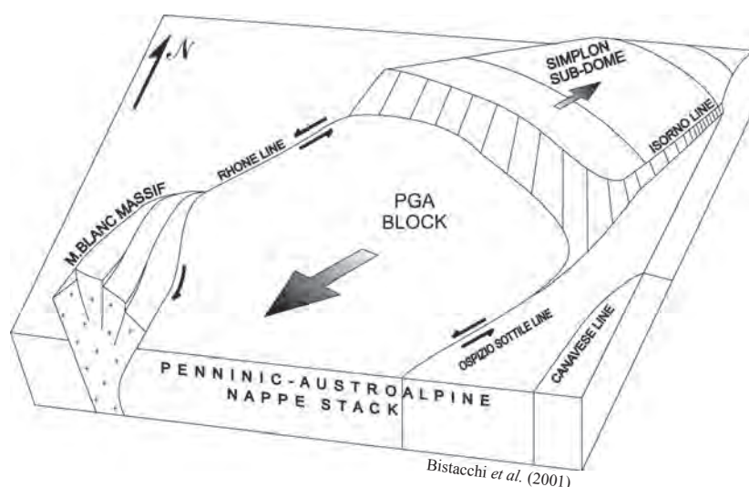
Figure V-1-6 : Modèle d'extrusion proposé par Bistacchi et al. (2001) entre le Mont Blanc et le dôme Lépointin.
