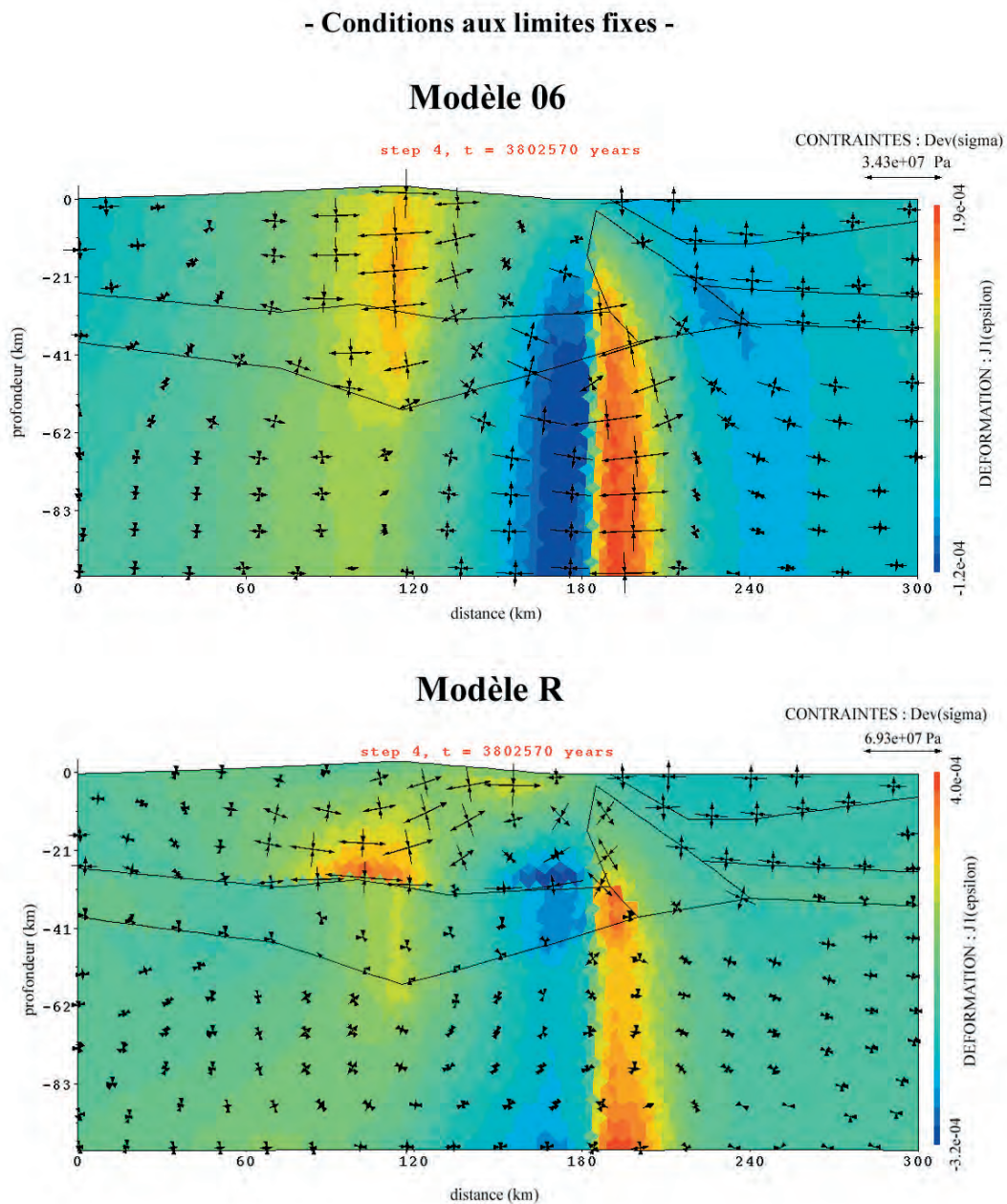
Figure II-2-2: Etat de déformation/contraintes calculé avec des conditions aux limites fixes. Tons jaune/rouge : déformation extensive, tons bleus : déformation compressive. Flèches : déviateurs de contraintes. Les 2 modèles présentés (R et 06) diffèrent par leurs caractéristiques rhéologiques (voir Tableau II-2-1).
