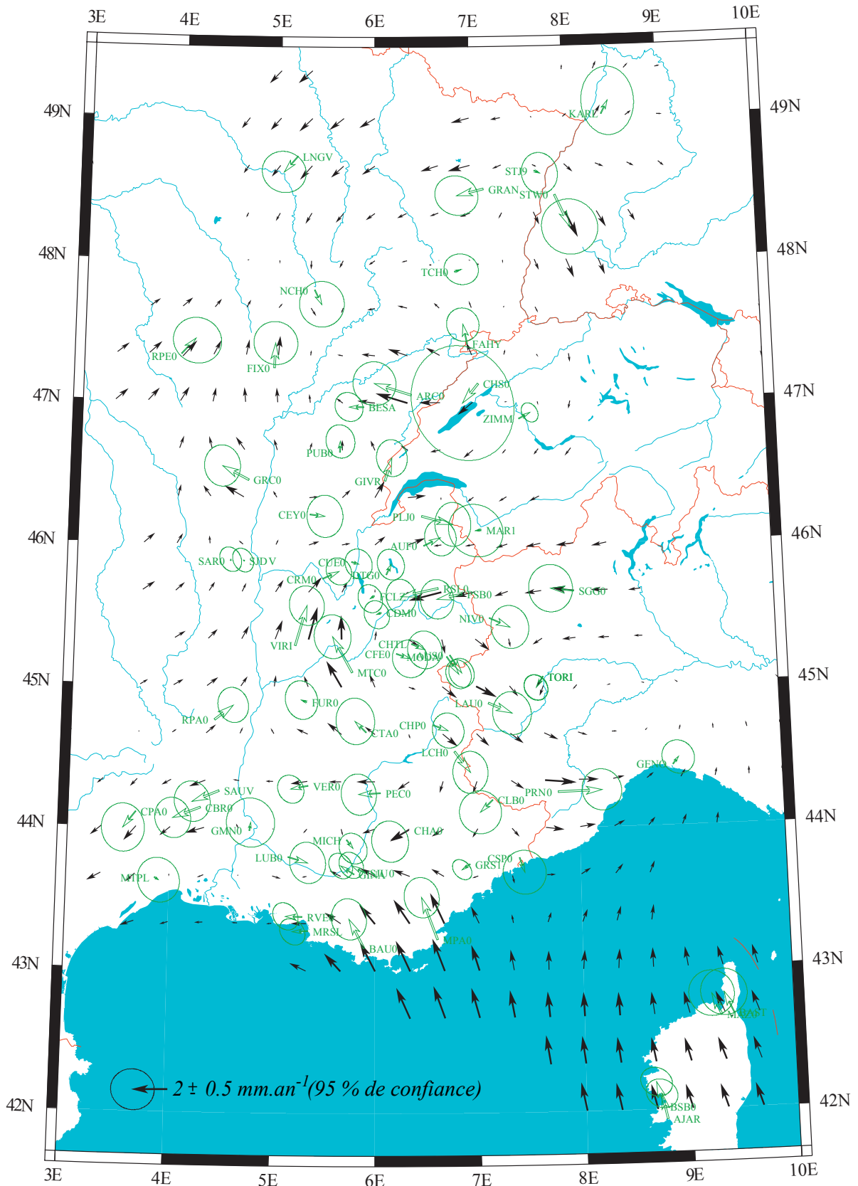
Figure III-1-3: Champs de vitesses GPS brutes (vert) et interpolée (noir) utilisés dans le calcul des taux de déformation. Noter la bonne correspondance entre les vitesses brutes et les vitesses interpolées.
