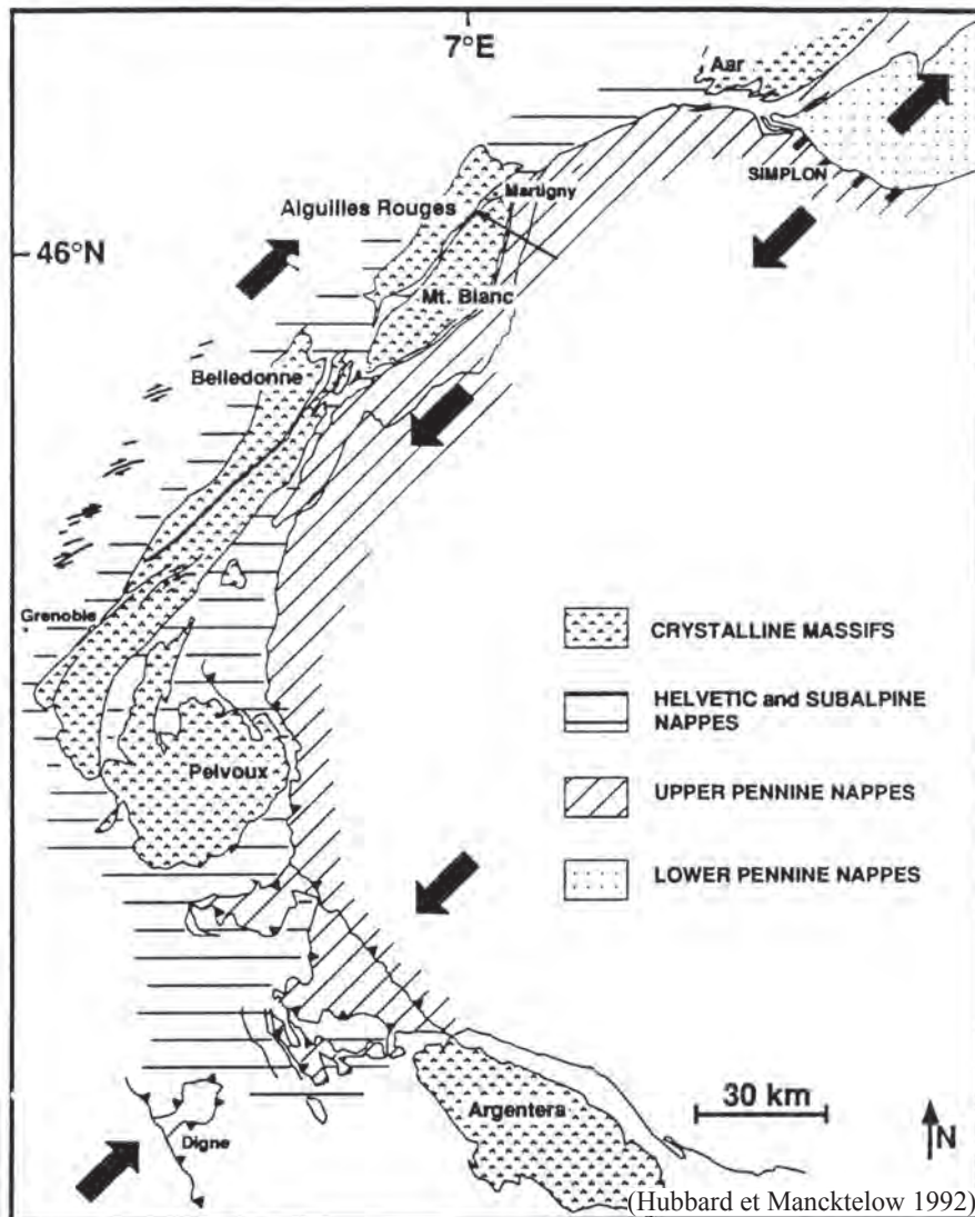
Figure V-1-5 : Modèle d'extrusion latérale proposé par Hubbard et Macktelow [1992]. Les quantités de mouvements et les âges de la déformation sont comparables entre la région du Simplon (extension) et les nappes de charriage du Sud-Ouest de l'arc Alpin.
