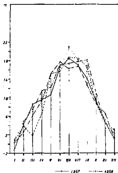
TEMPERATURE DE L'AIR
