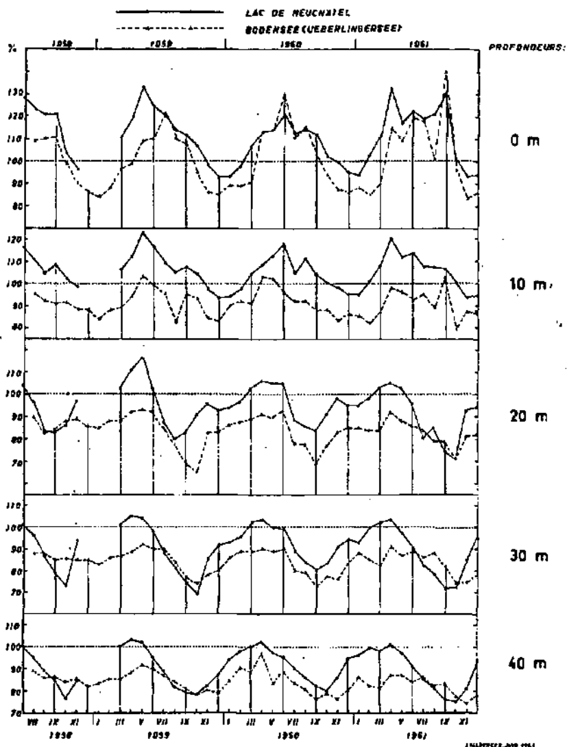
VARIATION MENSUELLE DE LA SATURATION D'OXYGENE, 1958-1961
