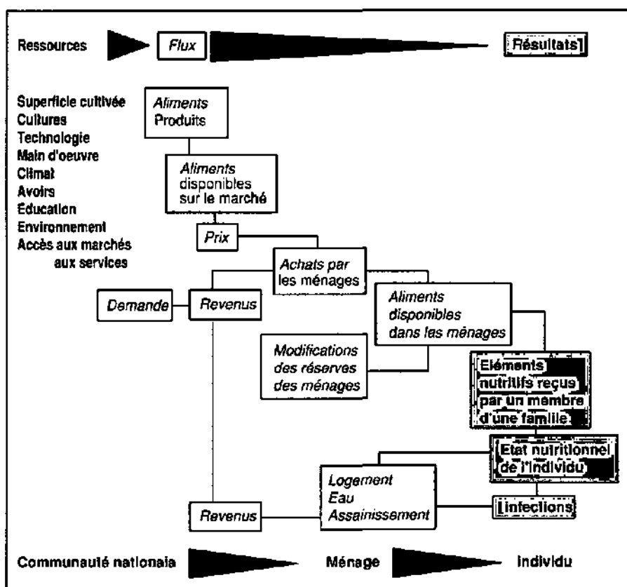
Fig. 30 :Relation entre les variables ressources, flux et état nutritionnel (d'après John B. et al. 1987)
