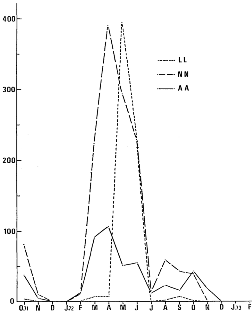
FIG. 1 : Échantillonnage mensuel des Tiques libres. LL : larves, NN : nymphes, AA : Adultes.
