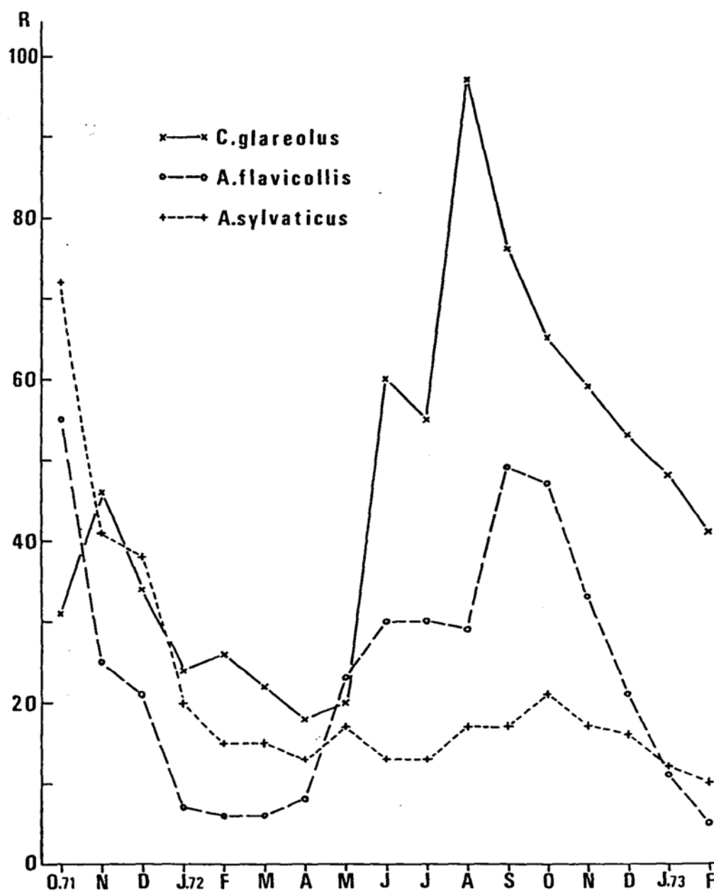
FIG. 2 : Densité de population des 3 espèces principales de Rongeurs (selon la méthode du calendrier des captures).
