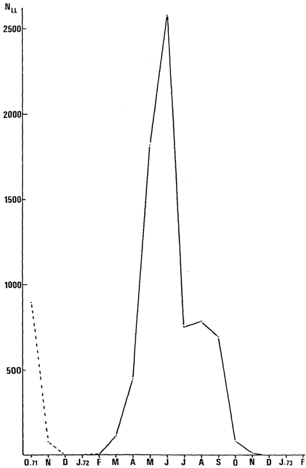
FIG. 3 : Estimations mensuelles du nombre total de larves fixées sur les Rongeurs. En pointillé : comptage, en trait continu : déparasitage (voir le texte).
