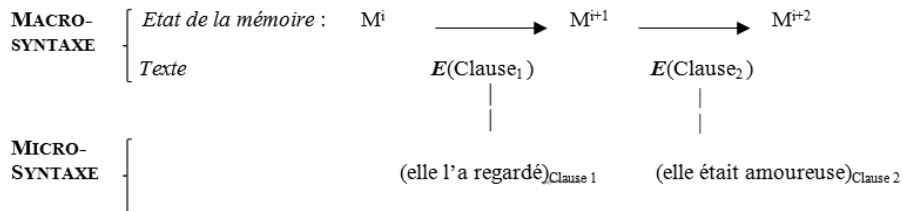
Figure 1 : L’articulation entre micro-syntaxe et macro-syntaxe (schéma inspiré de Berrendonner 2002)
