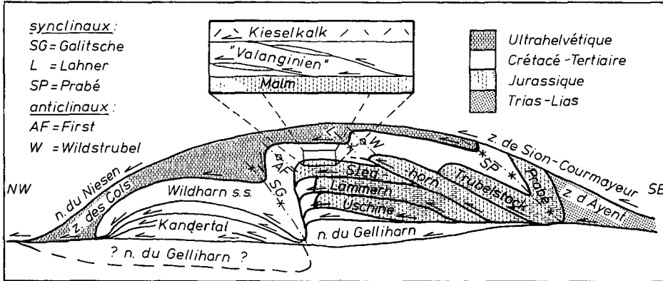
Fig. 5. Schéma des relations entre les différentes écailles de la nappe du Wildhorn. Les écailles jurassiques, décollées au niveau de l'Aalénien sont toutes en position normale sauf celle du Prabé. Le « Valanginien schisteux » (deuxième niveau de décollement), permet le comportement disharmonique des ensembles crétacés de la nappe du Wildhorn. Pour le grand pli du First et de Golitsche, dans le Crétacé de la nappe du Wildhorn, on perd les traces des plans axiaux anticlinale et synclinale, au front des écailles jurassiques. La nappe du Gellihorn sous-jacente peut être considérée comme écaille inférieure de la nappe du Wildhorn. Son extension au nord, sous les écailles du Kandertal, n'est pas connue.
