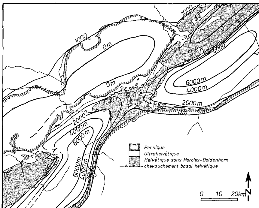
Fig. 10b. Isohypses du plan de chevauchement basal des nappes helvétiques (nappes du Wildhorn, des Diablerets, du Gellhorn et unités équivalentes); même principe de construction que pour la figure 10a. Au sud, la trace du chevauchement helvétique est jalonnée d'affleurements de Lias. Au nord, les isohypses sont dessinées en faisant l'hypothèse, que le chevauchement helvétique rejoint celui des Préalpes. La parallélisation des «massifs subalpins savoyards» avec les nappes des Diablerets et du Wildhorn (Douboux et al. 1982), crée un «genou» important dans la surface du plan de chevauchement basal au SW du massif des Aiguilles-Rouges, qu'il reste à expliquer. Une solution minimale est représentée par les isohypses au-dessus des massifs cristallins tandis qu'une dépression minimale est proposée sous les Préalpes et les lacs de Thoune et de Brienz.
