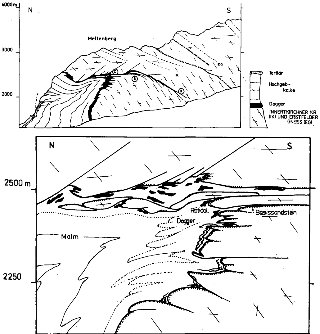
Abb. 7 Profile des Mettenberges (nach eigenen Feldaufnahmen). Abb. 7a: Gesamtprofil. Abb. 7b: Ausschnitt c, Abb. 7a.
