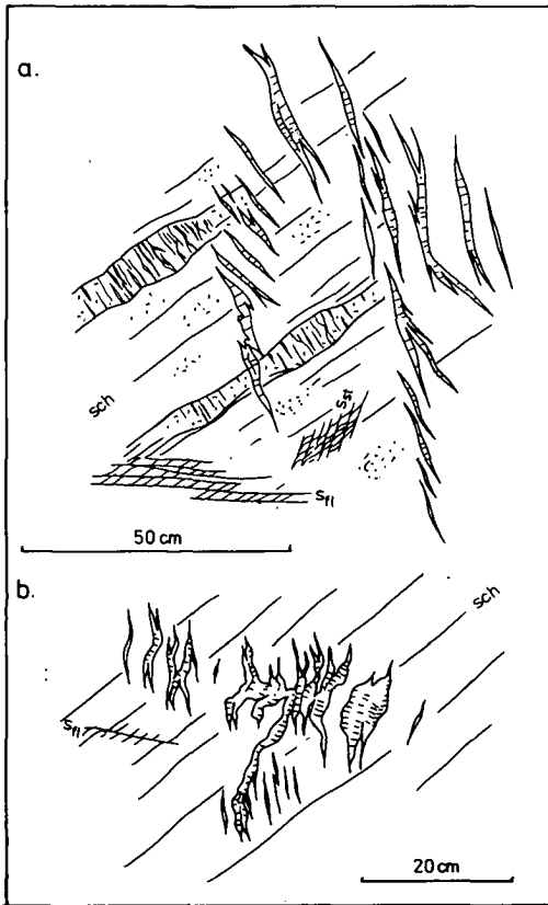
Abb. 2 Gefüge im Erstfelder Gneis, Unterer Grindelwaldgletscher. - Abkürzungen: Z_1 Zerrklüfte in en-échelon-Anordnung, Z_2 Zerrissen in kompetenten Lagen, sch Schieferung und Gneisbänderung, sfl flache Schieferflächen mit dextralem Schersinn, sst steile Schieferflächen mit sinistralen Schersinn. Abb. 2a zeigt die beiden Arten von Zerrklüften, während Abb. 2b teilweise leicht verfaltete Zerrklüfte aus einer Scherzone wiedergibt.
