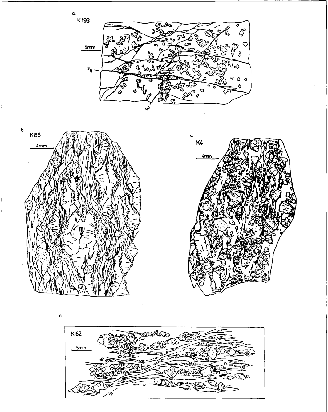
Abb. 12 Ausgewählte Mikrostrukturen. - Signaturen: Quarz punktiert, Kalifeldspat randlich punktiert, Grundmasse gestrichelt, Biotit ausgezogene Striche, Karbonat- rhomboeder schwarz. a: Spröd verformtes aplitisches Gestein. Nebst den Bruchflächen sind nur die Umrisse grösserer Quarze gezeichnet. b: spröd-duktil verformtes kalifeldspatreiches Gestein. c: spröd-duktil verformtes biotitreiches Gestein. d: phyllitisches Gestein mit stark fragmentierten Quarzen. S_{II} ist ein Scherband.
