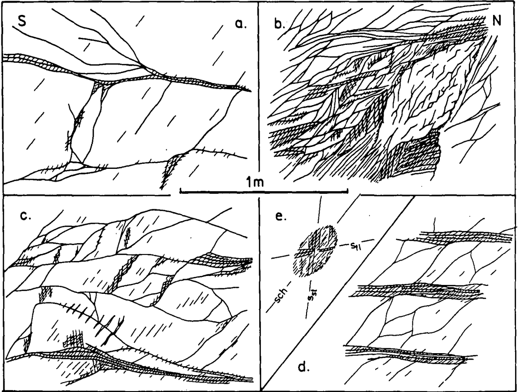
Abb. 4 Gefüge und Strukturen aus vier unterschiedlich verformten Bereichen des Innerkirchner Kristallins. Die angegebenen R_s -Werte sind Achsenverhältnisse der Verformungsellipse der Sedimente am Sediment-Kristallin-Kontakt abgeschätzt (KAMMER, 1985).
